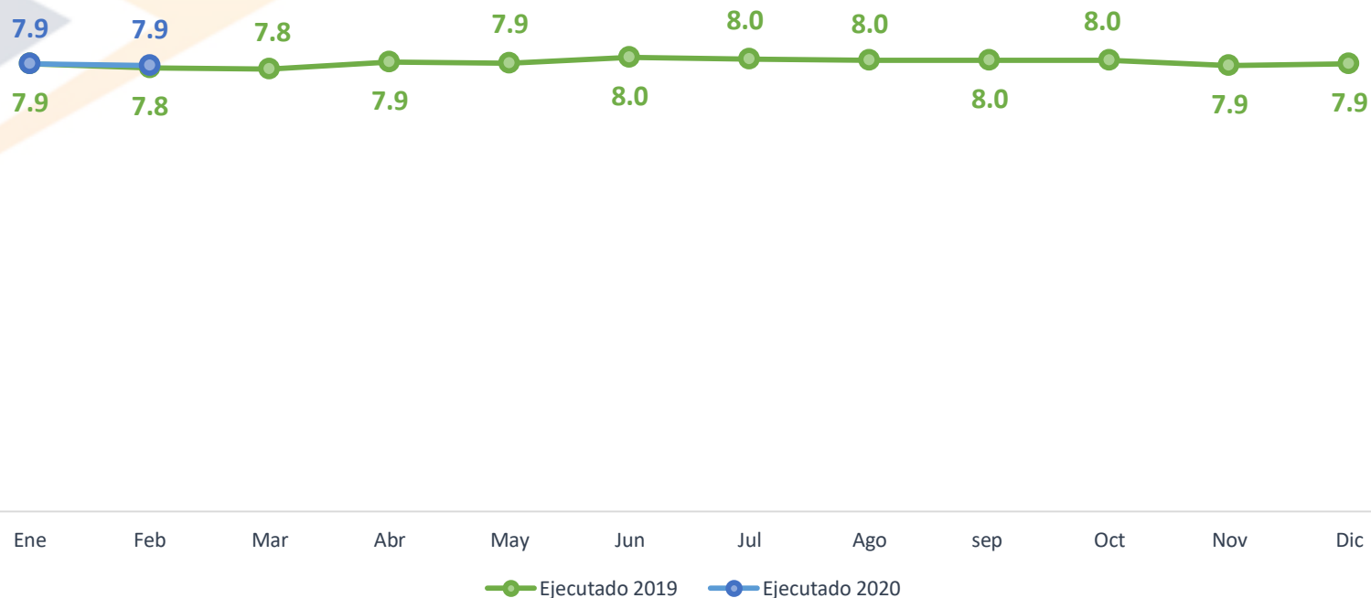
Precio Medio de Venta de Energía Total EDE's 2020 - 2019 RD$/kWh
