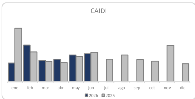
Figura 14. CAIDI
