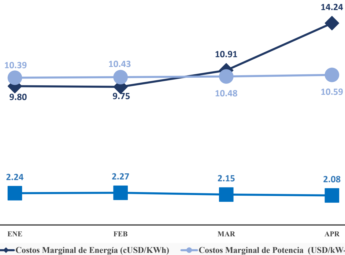
Costos Marginales de Energía, Potencia y Derecho de Conexión Unitario enero-abril 2026 (cUSD/kWh y USD/kW-período )
