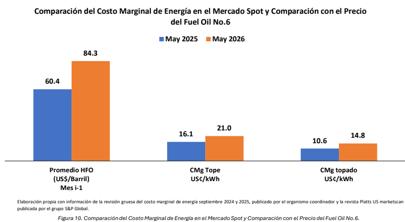
Figura 10. Comparación del Costo Marginal de Energía en el Mercado Spot y Comparación con el Precio del Fuel Oil No.6.
