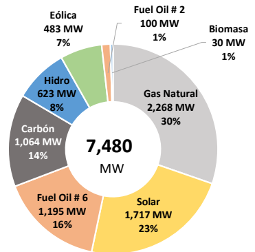
Capacidad Instalada Nominal por Fuente Primaria - mayo 2026
