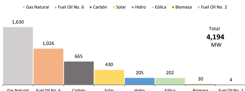
Disponibilidad Promedio del SENI por Fuente Primaria - mayo 2026
