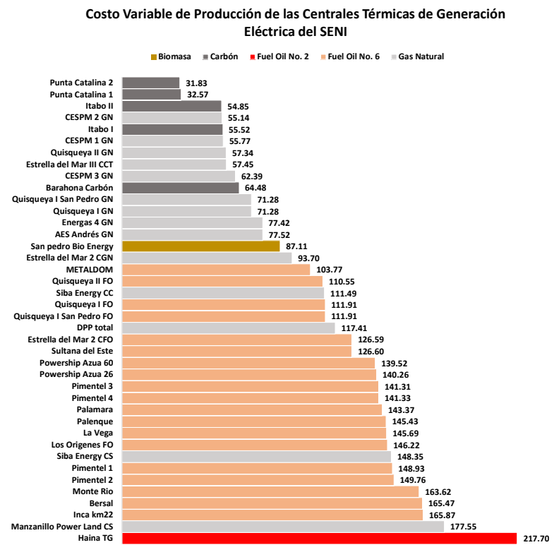
Figura 9. Costo Variable de Producción de las Centrales Térmicas de Generación Eléctrica del SENI.
