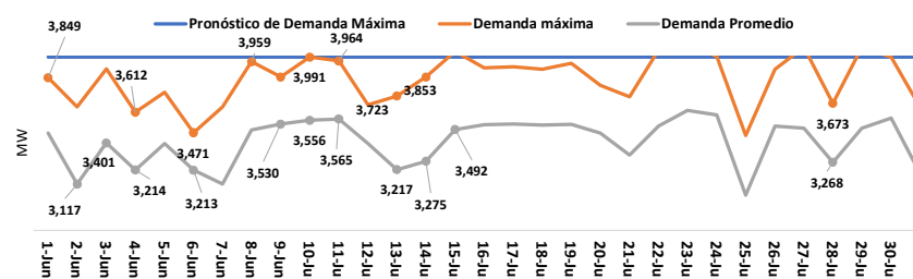
Figura 5. Evolución Demanda de Potencia del SENI - mayo 2026.
