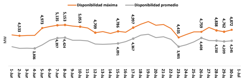
Evolución Disponibilidad Centrales Generación del SENI - mayo 2026
