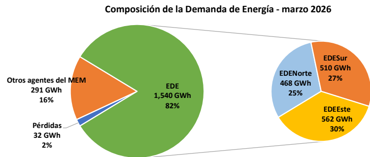
Figura 4. Composición de la Demanda de Energía - marzo 2026
