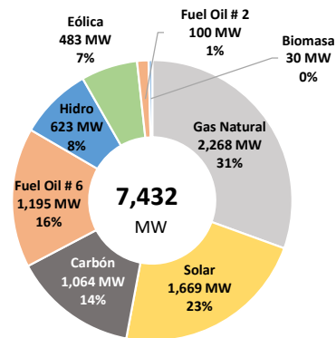
Capacidad Instalada Nominal por Fuente Primaria - marzo 2026
