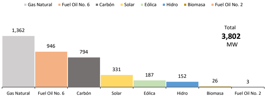
Disponibilidad Promedio del SENI por Fuente Primaria - marzo 2026
