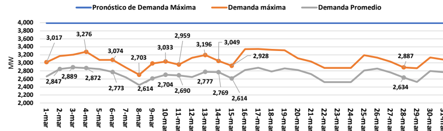
Figura 5. Evolución Demanda de Potencia del SENI - marzo 2026.
