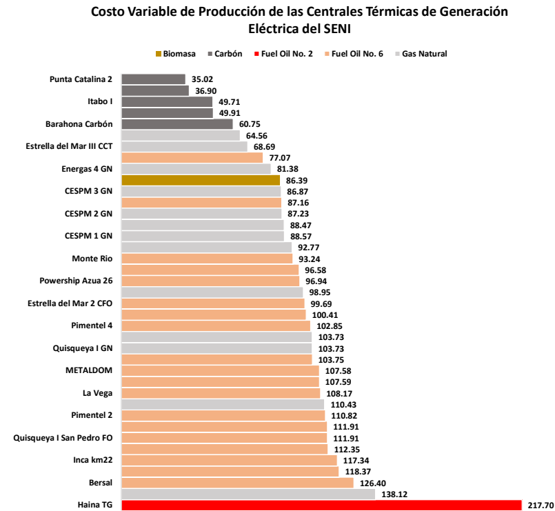
Figura 9. Costo Variable de Producción de las Centrales Térmicas de Generación Eléctrica del SENI.
