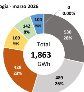
Generación de Energía Eléctrica por Tecnología - marzo 2026
