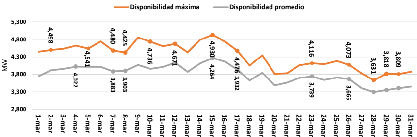
Evolución Disponibilidad Centrales Generación del SENI - marzo 2026
