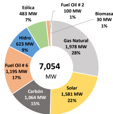
Capacidad Instalada Nominal por Fuente Primaria - enero 2026
