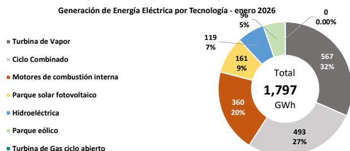
Figura 7. Generación de Energía Eléctrica por Tecnología - enero 2026
