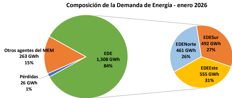
Figura 4. Composición de la Demanda de Energía - enero 2026
