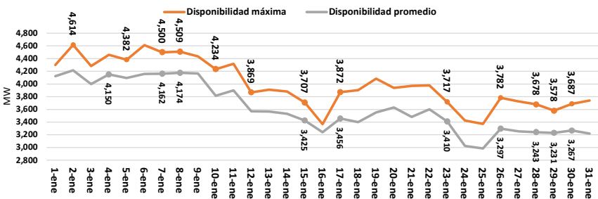
Evolución Disponibilidad Centrales Generación del SENI - enero 2026
