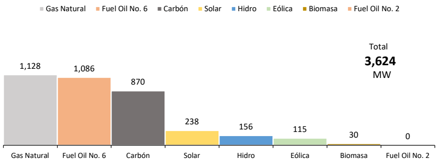
Disponibilidad Promedio del SENI por Fuente Primaria - enero 2026
