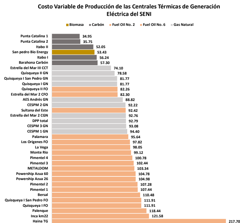
Figura 9. Costo Variable de Producción de las Centrales Térmicas de Generación Eléctrica del SENI.
