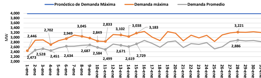
Figura 5. Evolución Demanda de Potencia del SENI - enero 2026.
