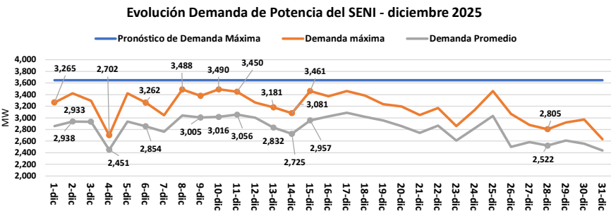
Figura 5. Evolución Demanda de Potencia del SENI - diciembre 2025.
