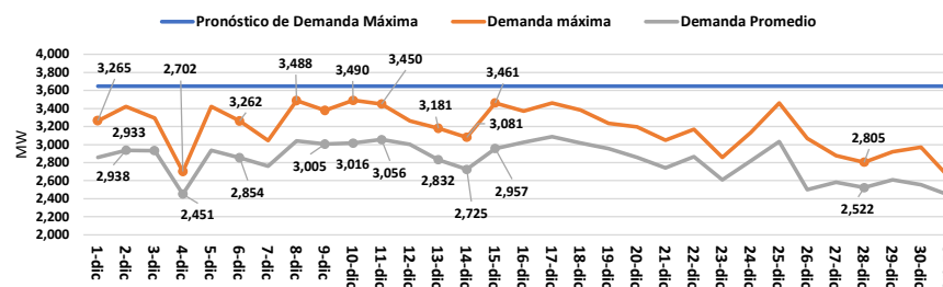
Figura 5. Evolución Demanda de Potencia del SENI - diciembre 2025.
