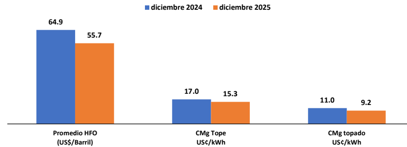
Figura 10. Comparación del Costo Marginal de Energía en el Mercado Spot y Comparación con el Precio del Fuel Oil No.6.
