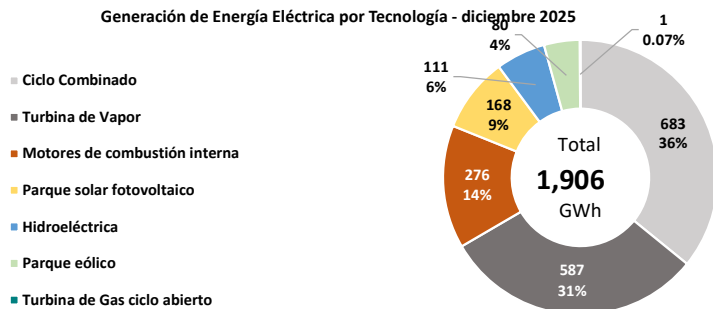
Figura 7. Generación de Energía Eléctrica por Tecnología - diciembre 2025.
