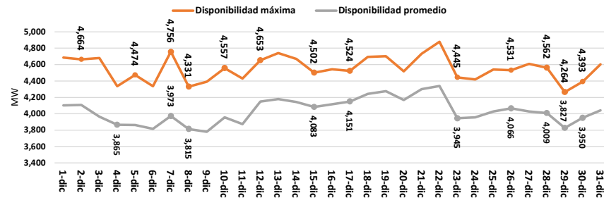
Evolución Disponibilidad Centrales Generación del SENI - diciembre 2025
