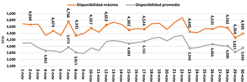
Evolución Disponibilidad Centrales Generación del SENI - noviembre 2025
