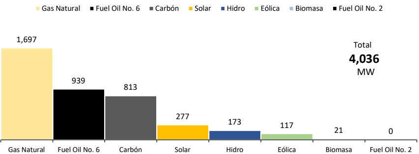
Disponibilidad Promedio del SENI por Fuente Primaria - noviembre 2025
