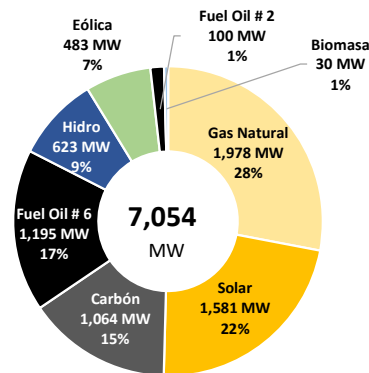
Capacidad Instalada Nominal por Fuente Primaria - noviembre 2025
