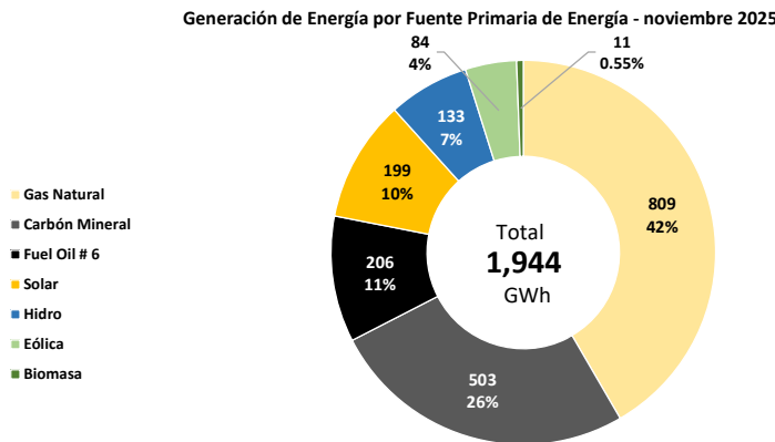
Figura 6. Generación de Energía por Fuente Primaria de Energía - noviembre 2025
