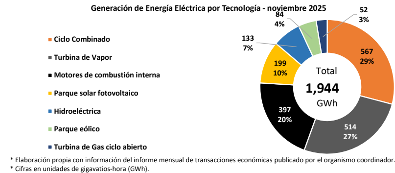
Figura 7. Generación de Energía Eléctrica por Tecnología - noviembre 2025.
