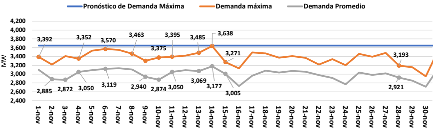
Figura 5. Evolución Demanda de Potencia del SENI - noviembre 2025.
