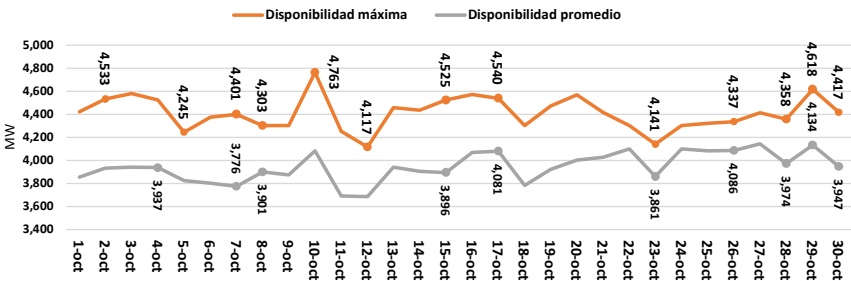
Evolución Disponibilidad Centrales Generación del SENI - octubre 2025
