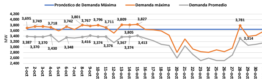
Figura 5. Evolución Demanda de Potencia del SENI - octubre 2025.
