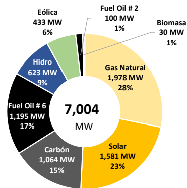
Capacidad Instalada Nominal por Fuente Primaria - octubre 2025
