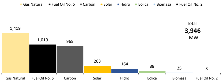
Disponibilidad Promedio del SENI por Fuente Primaria - octubre 2025
