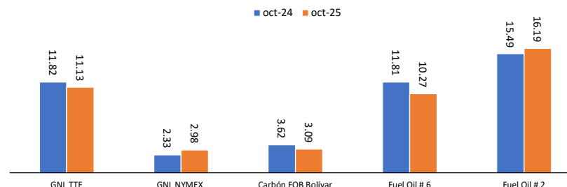
Figura 8. Comparación Precios Combustibles Mercados Internacionales - octubre 2024 vs. 2025
