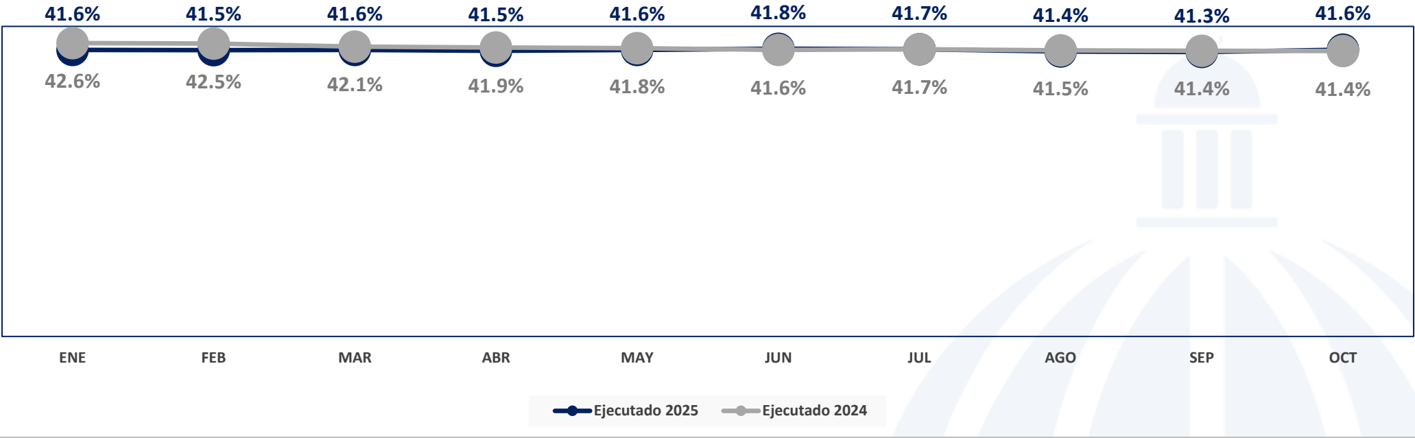
Comparativo Índice Recuperación Energía - Año Móvil (%)
