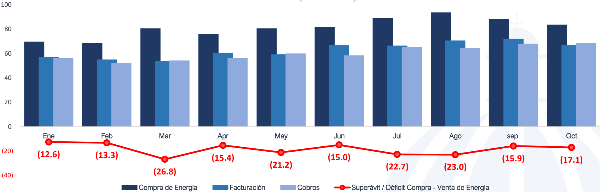
Factura de Compra - Facturación - Cobros Edenorte enero-octubre 2025 (MM USD)
