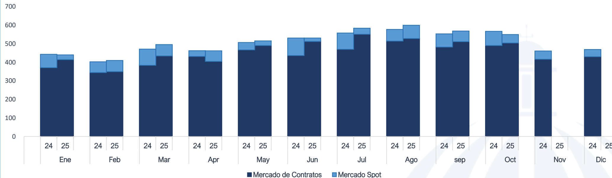
Compra de Energía por Mercado Edenorte enero-octubre 2025/ enero-octubre 2024 (GWh)
