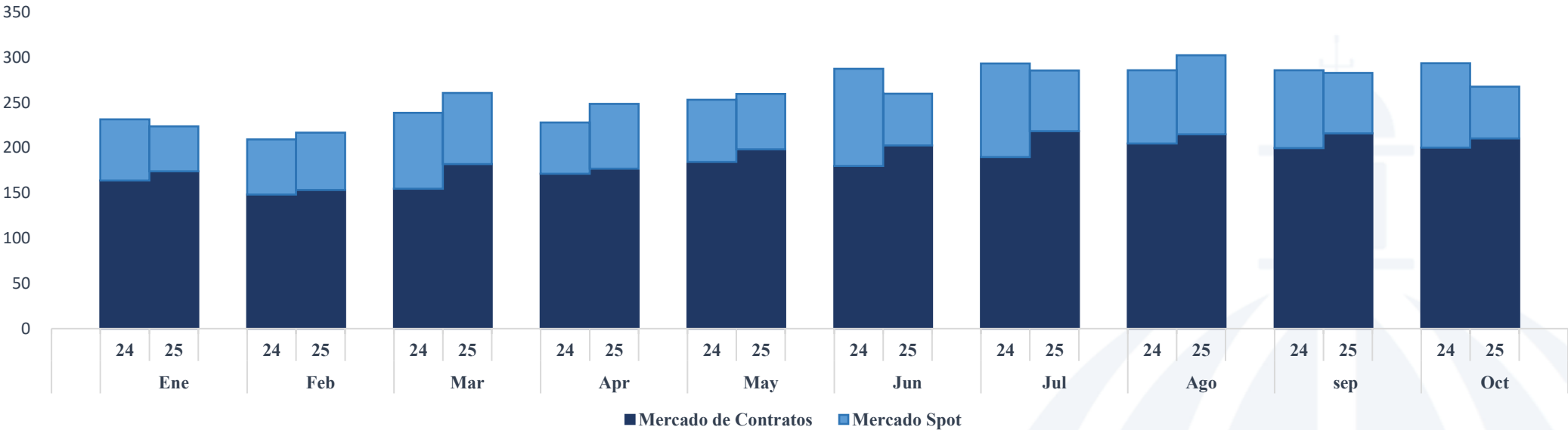
Factura Compra de Energía por Mercado Total EDE's enero-octubre 2025/ enero-octubre 2024 (USD MM)
