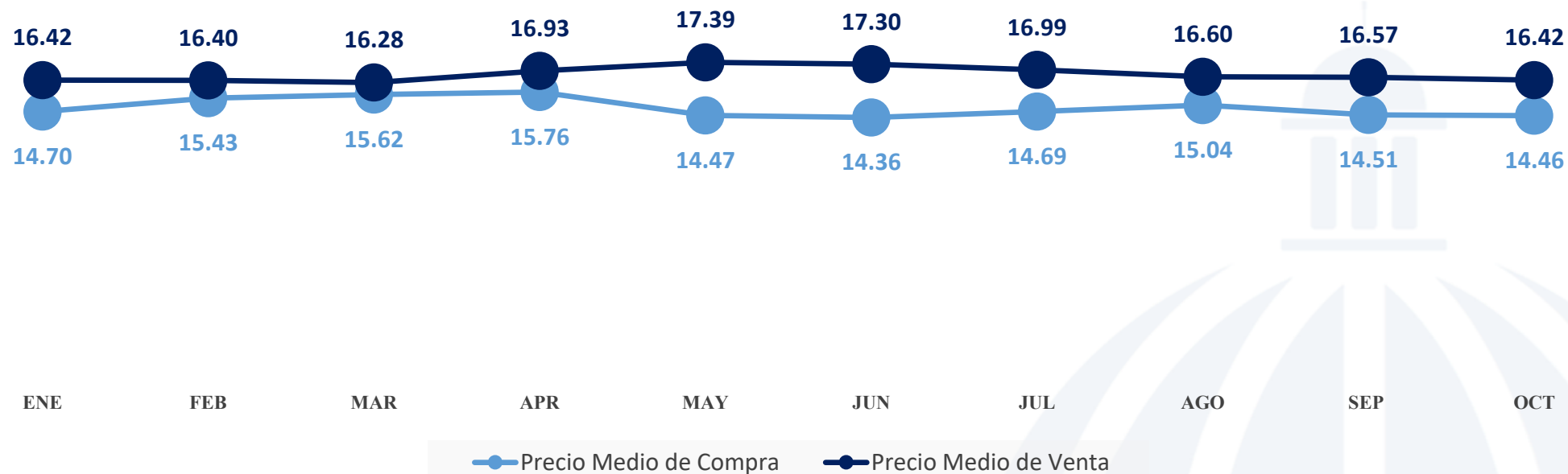
Precio Medio de Compra y Venta de Energía Edesur enero-octubre 2025 (USDCents/kWh)
