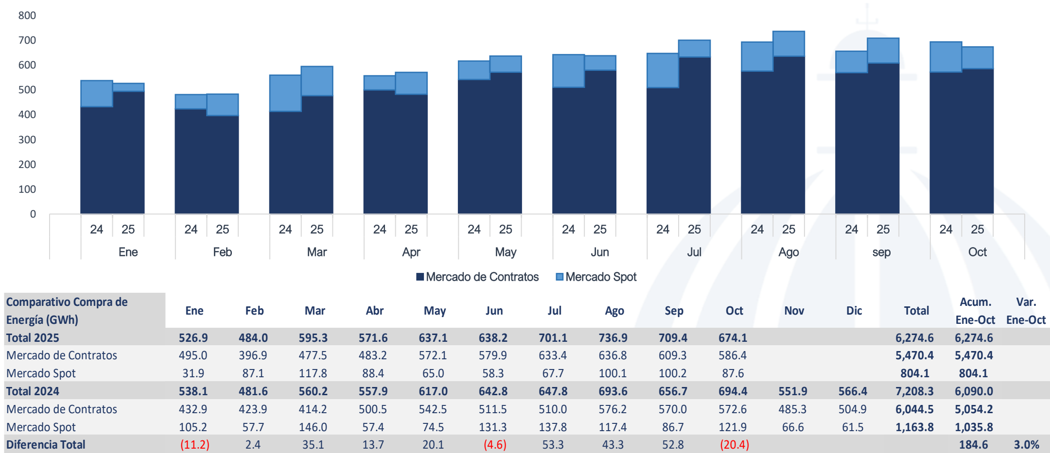
Compra de Energía por Mercado Edeeste enero-octubre 2025- enero-octubre 2024 (GWh)
