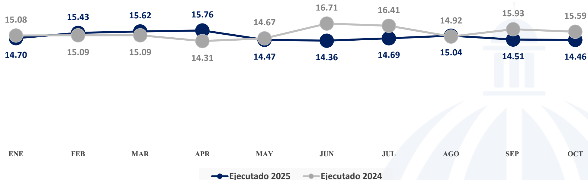
Precio Medio de Compra de Energía Edesur enero-octubre 2025/ enero-octubre 2024 (cUSD/kWh)
