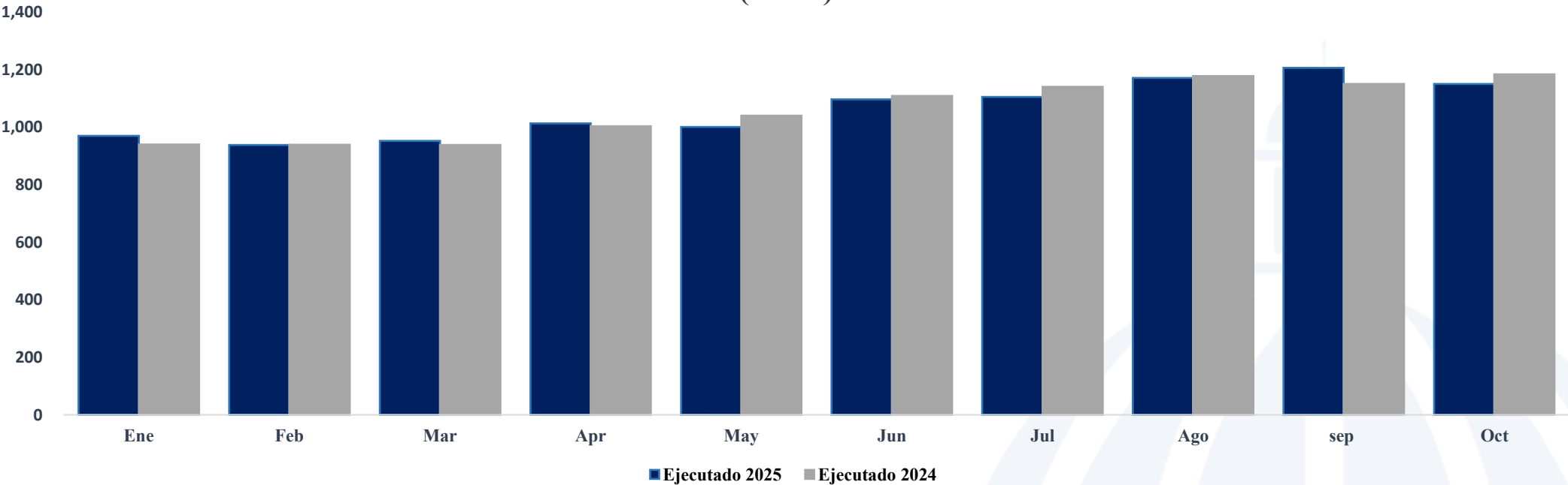
Energía Facturada Total EDE's enero-octubre 2025/ enero-octubre 2024 (GWh)
