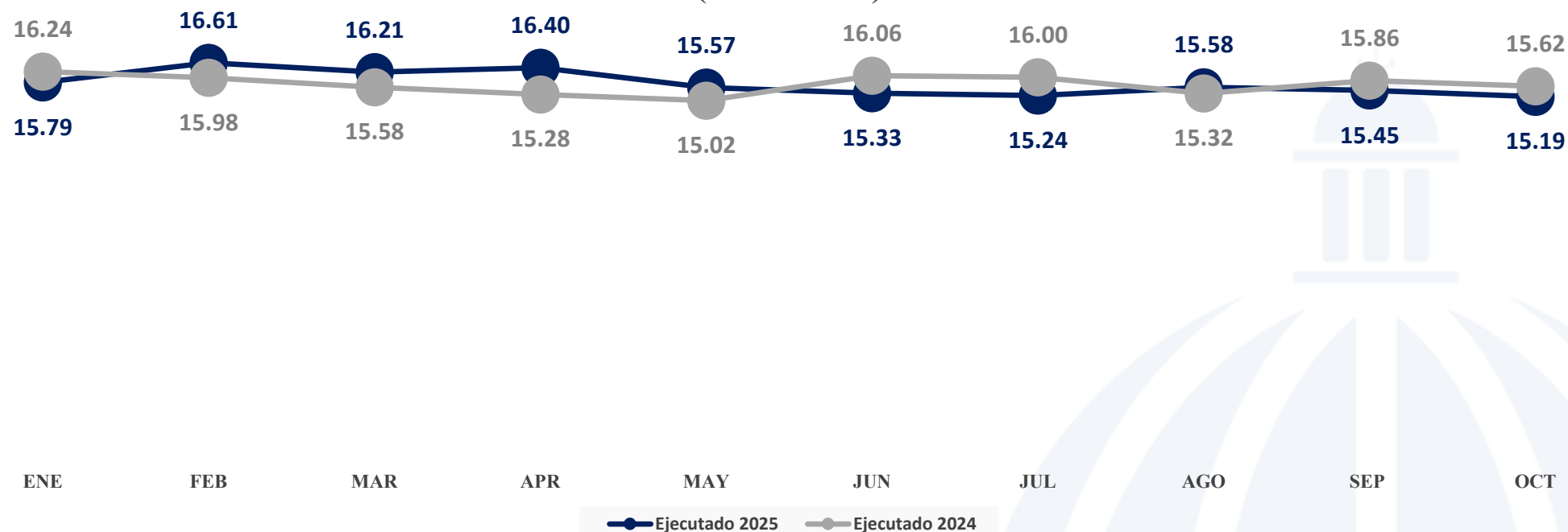
Precio Medio de Compra de Energía Edenorte enero-octubre 2025/ enero-octubre 2024 (cUSD/kWh)
