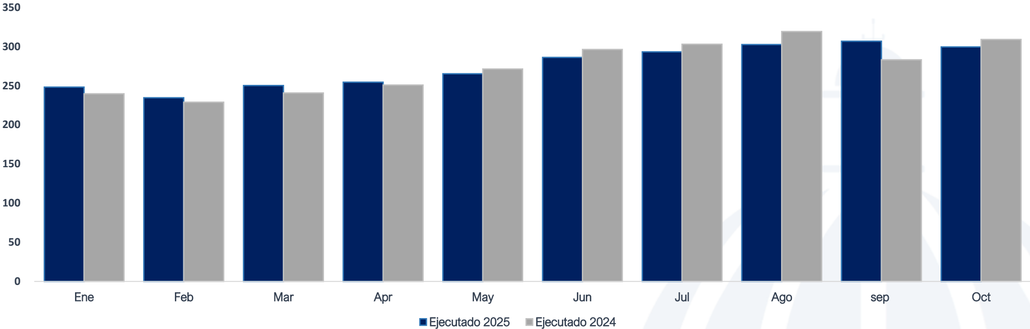
Energía Facturada Edeeste enero-octubre 2025- enero-octubre 2024 (GWh)
