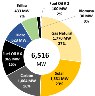
Capacidad Instalada Nominal por Fuente Primaria - septiembre 2025
