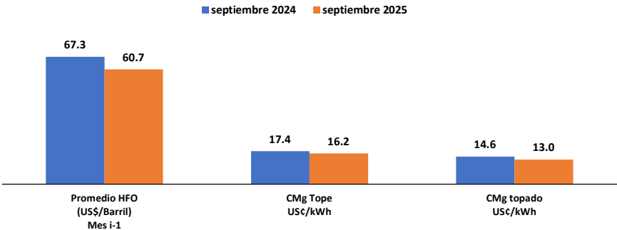
Comparación del Costo Marginal de Energía en el Mercado Spot y Comparación con el Precio del Fuel Oil No.6
