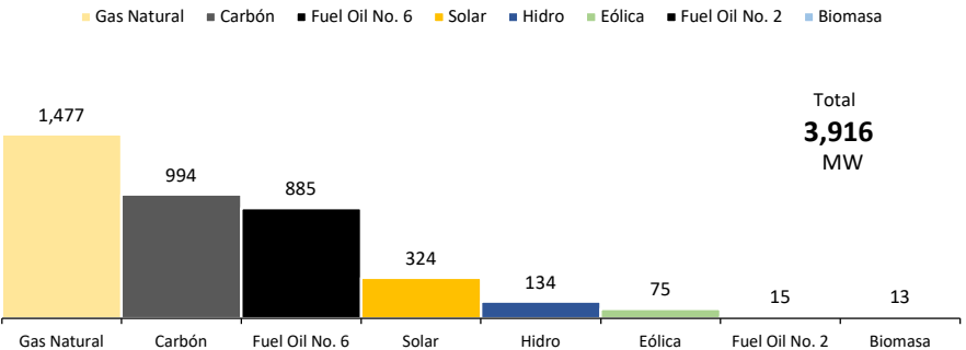
Disponibilidad Promedio del SENI por Fuente Primaria - septiembre 2025
