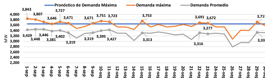
Figura 5. Evolución Demanda de Potencia del SENI - septiembre 2025.
