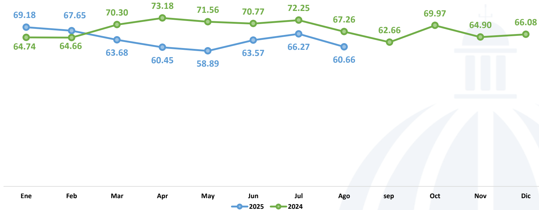
Precio de Combustible Fuel Oil #6 enero-agosto 2025/ enero-agosto 2024 (US$/BBL)
