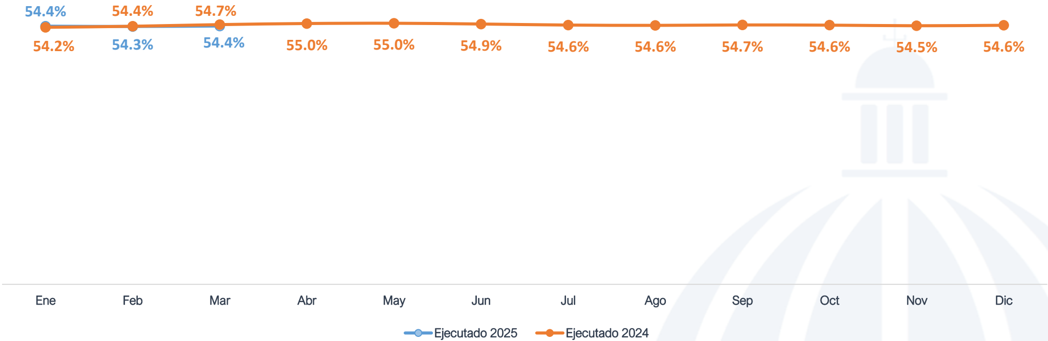
Pérdidas - Año Móvil Edeeste 2025 – 2024 Valores Porcentuales
