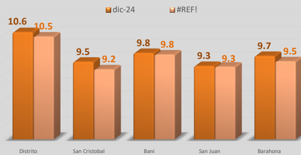
Monómico EDESur (RD$/kWh)
