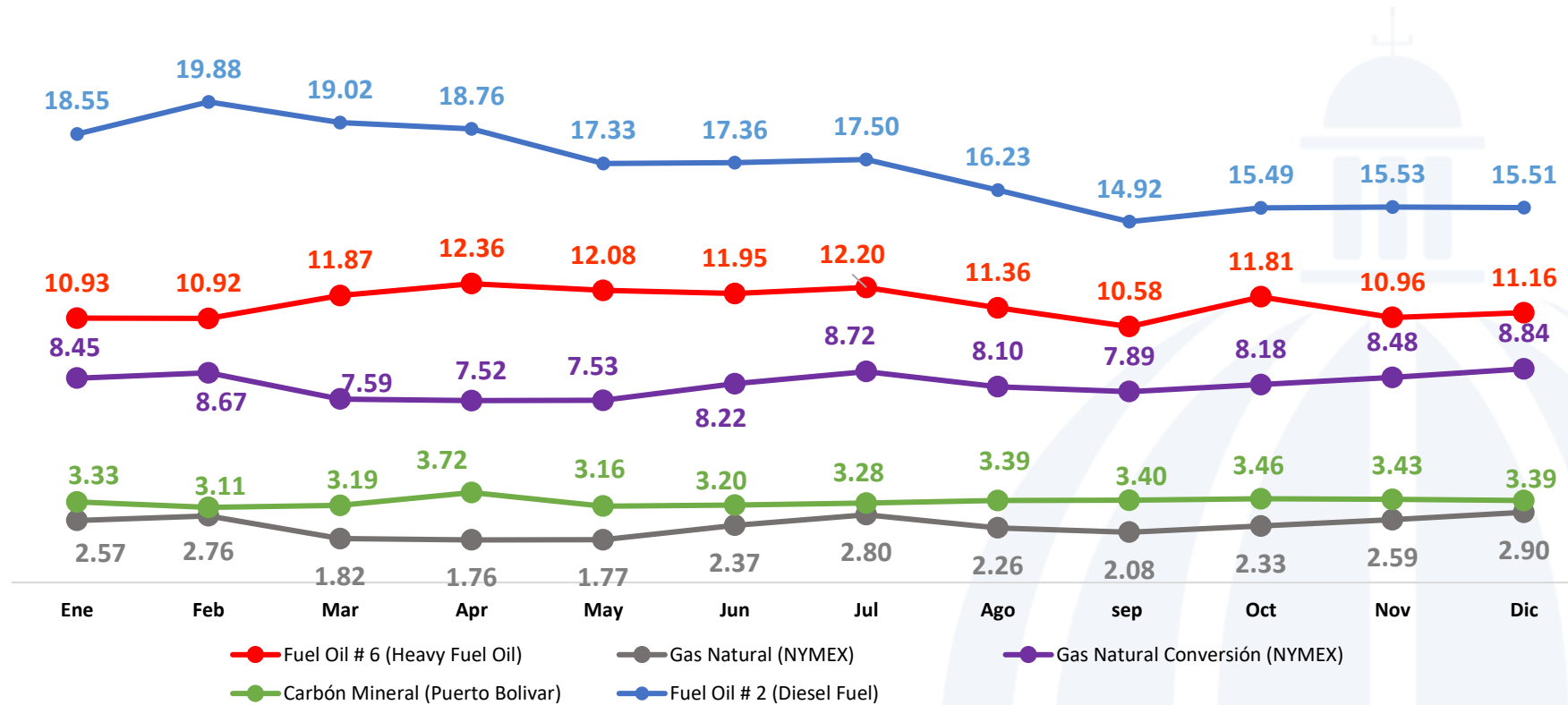
Precio de Combustibles enero-diciembre 2024 (US$/MMBTU)
