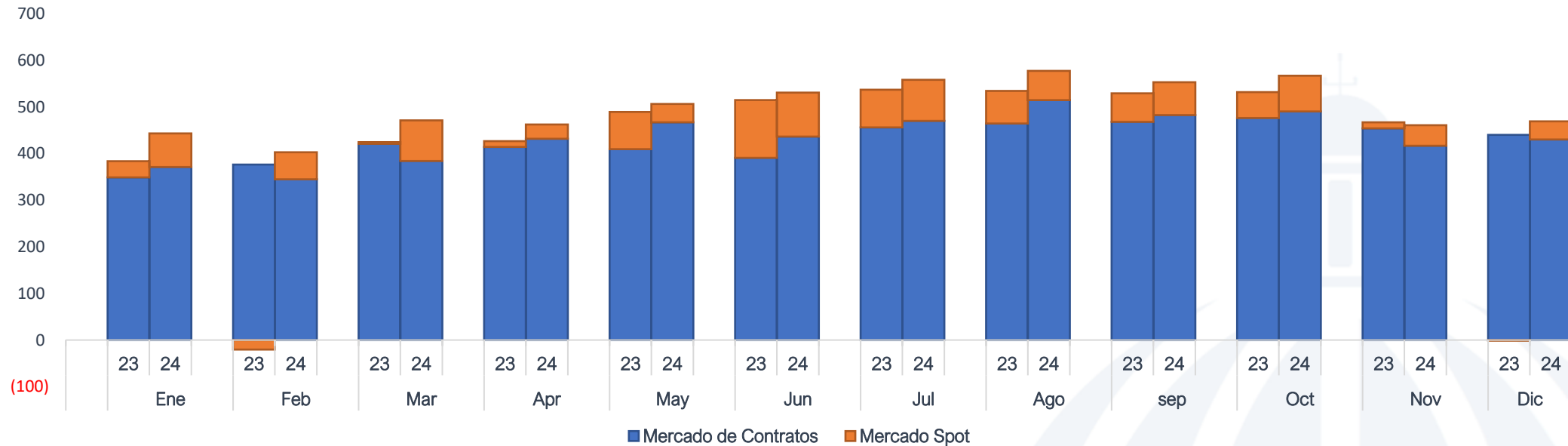
Compra de Energía por Mercado Edenorte enero-diciembre 2024/ enero-diciembre 2023 (GWh)
