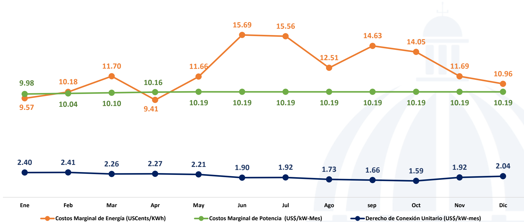
Costos Marginales de Energía, Potencia y Derecho de Conexión Unitario enero-diciembre 2024 (USCents/kWh y US$/kW-período de)
