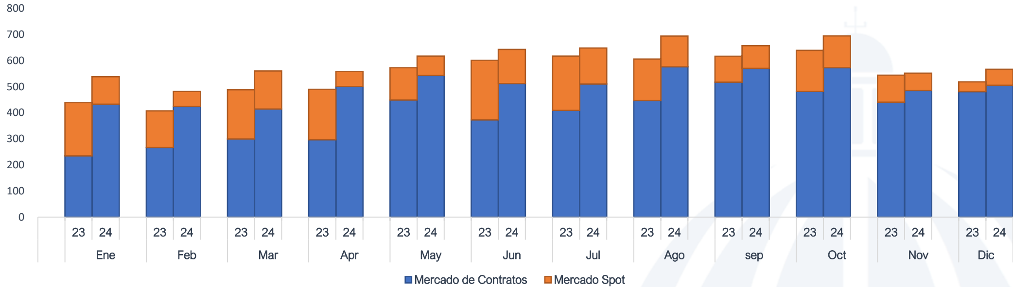
Compra de Energía por Mercado Edeeste enero-diciembre 2024- enero-diciembre 2023 (GWh)
