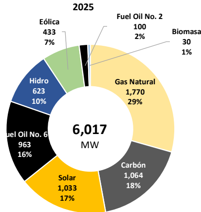
Matriz de capacidad nominal instalada - enero 2025
