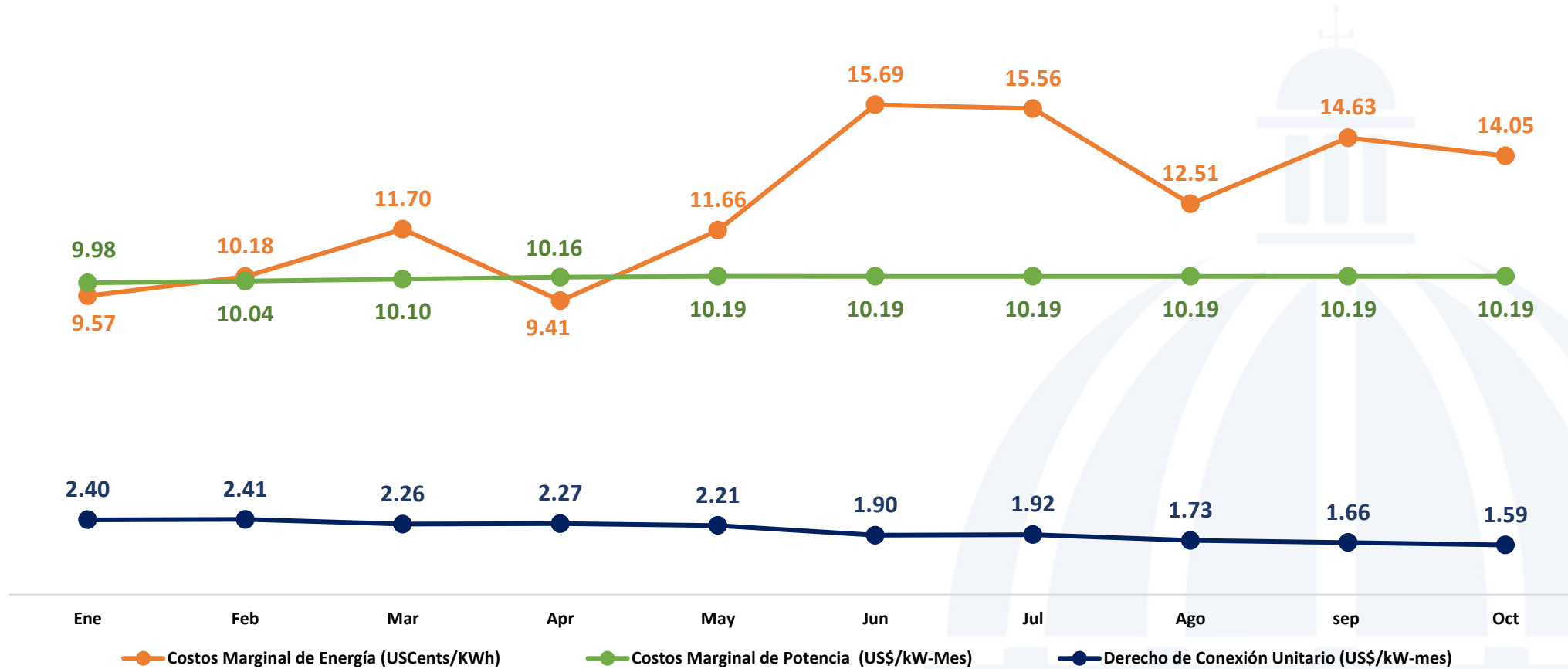
Costos Marginales de Energía, Potencia y Derecho de Conexión Unitario enero-octubre 2024 (USCents/kWh y US$/kW-período de)
