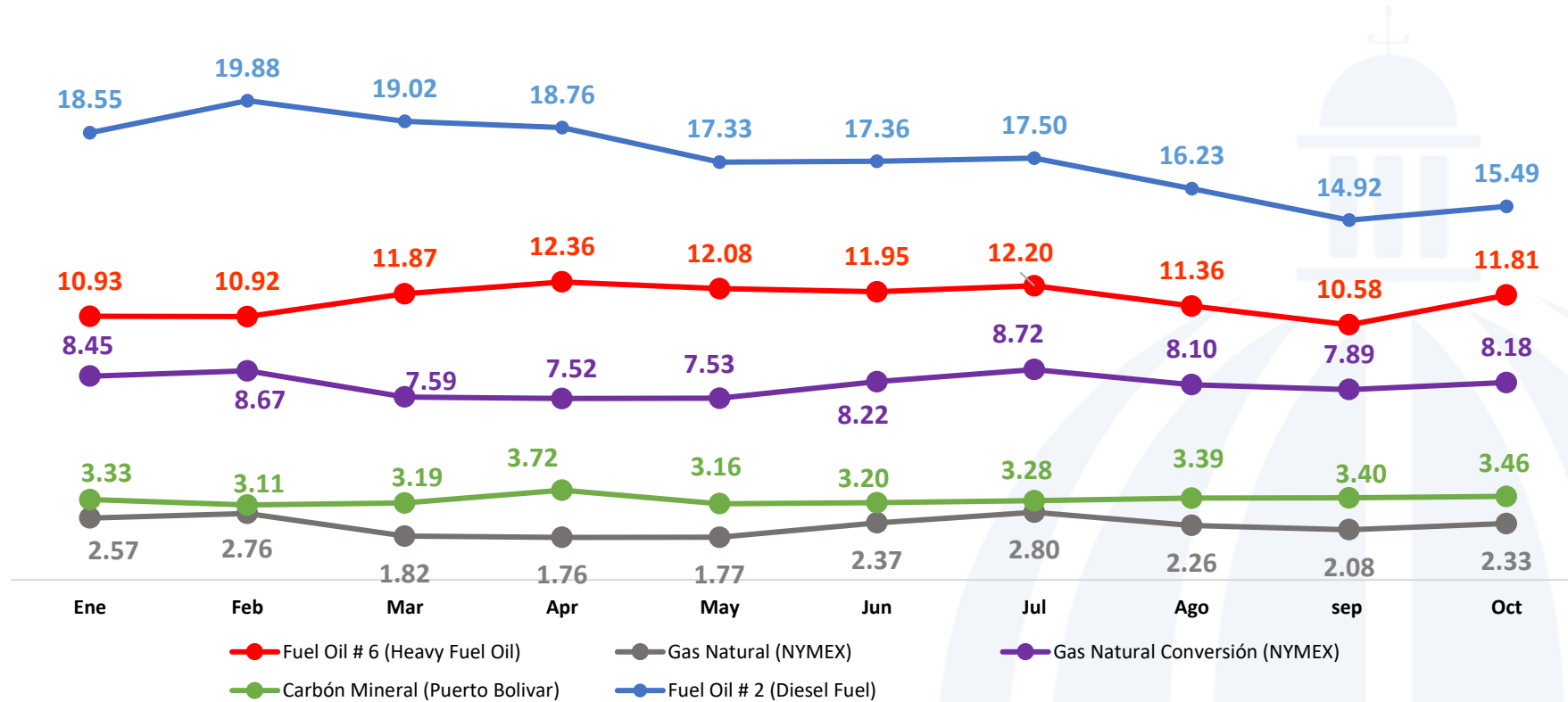
Precio de Combustibles enero-octubre 2024 (US$/MMBTU)
