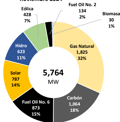
Matriz de capacidad nominal instalada - noviembre 2024
