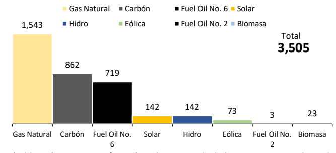
Disponibilidad promedio del SENI por combustible - noviembre 2024
