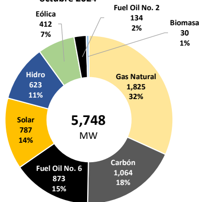
Matriz de capacidad nominal instalada - octubre 2024
