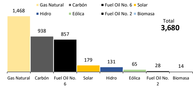
Disponibilidad promedio del SENI por combustible - octubre 2024
