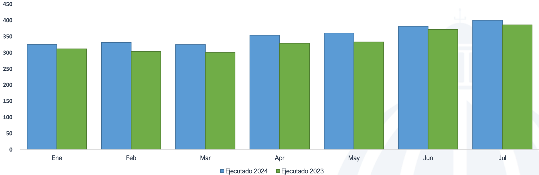
Energía Facturada Edenorte enero-julio 2024/ enero-julio 2023 (GWh)
