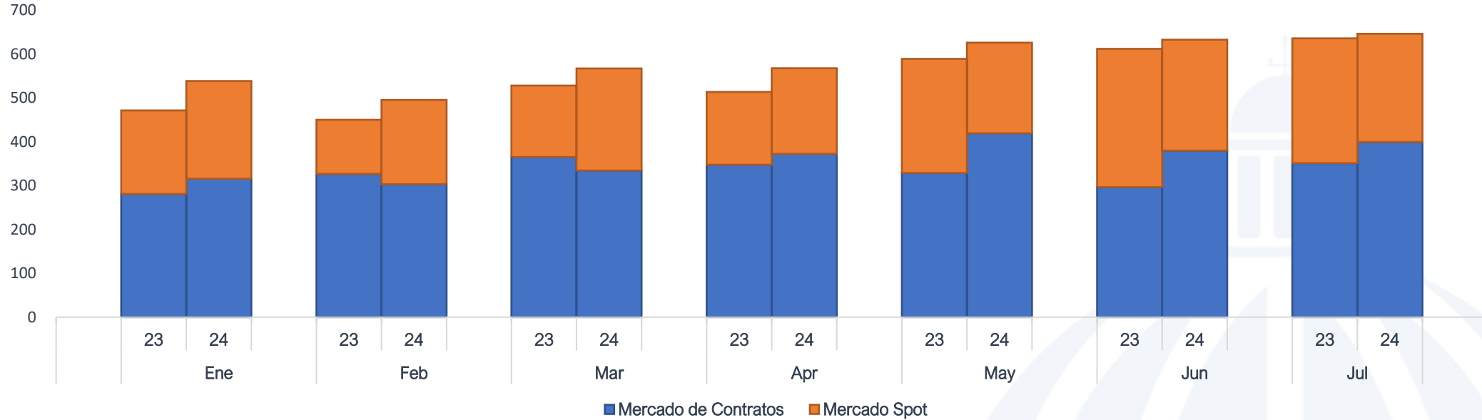
Compra de Energía por Mercado Edesur enero-julio 2024/ enero-julio 2023 (GWh)
