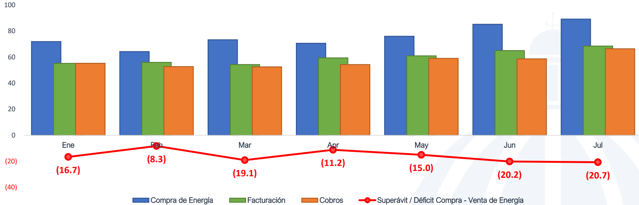
Factura de Compra - Facturación - Cobros Edenorte enero-julio 2024 (US$ MM)
