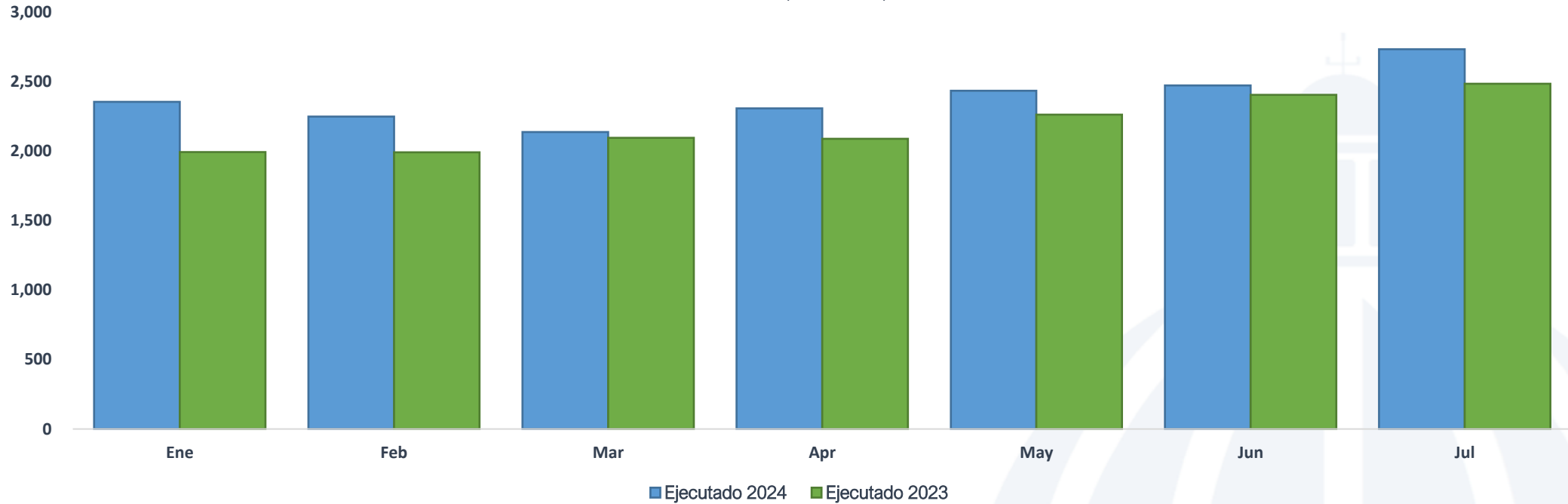
Comparativo Cobros Total Edeeste enero-julio 2024- enero-julio 2023 (RD$ MM)
