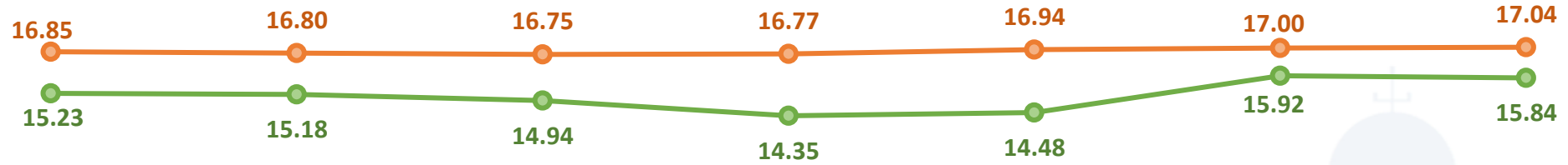
Precio Medio de Compra y Venta de Energía Total EDE's enero-julio 2024 (USCents/kWh)
