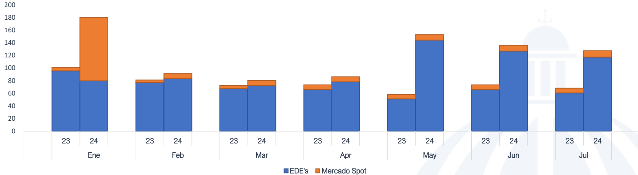
Energía Facturada EGEHID enero-julio 2024/ enero-julio 2023 (GWh)
