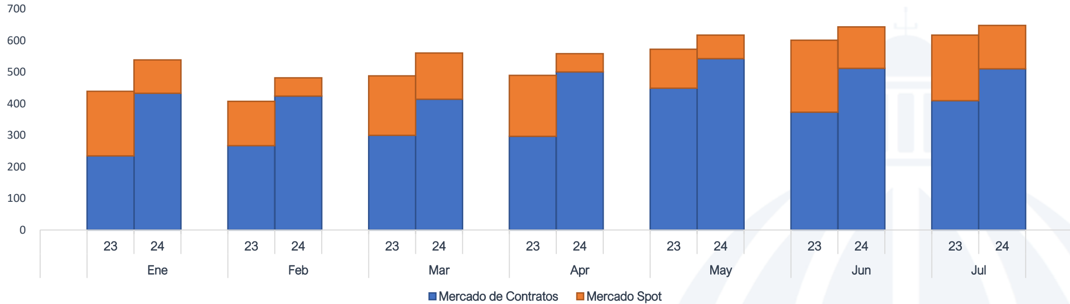
Compra de Energía por Mercado Edeeste enero-julio 2024- enero-julio 2023 (GWh)
