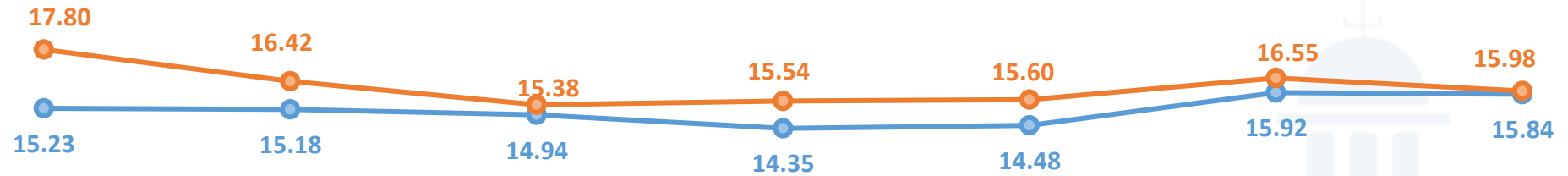
Precio Medio de Compra de Energía Total EDE's enero-julio 2024/ enero-julio 2023 (USCents/kWh)
