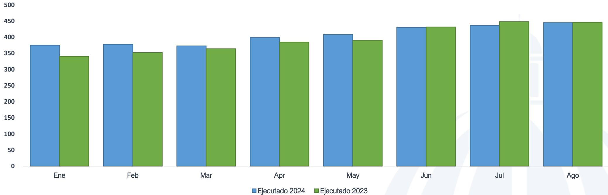
Energía Facturada Edesur enero-agosto 2024/ enero-agosto 2023 (GWh)
