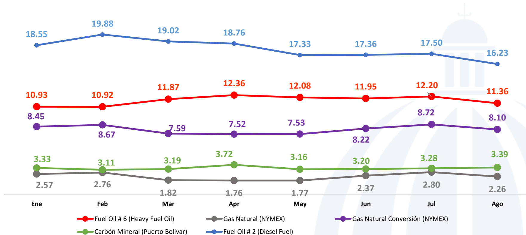
Precio de Combustibles enero-agosto 2024 (US$/MMBTU)
