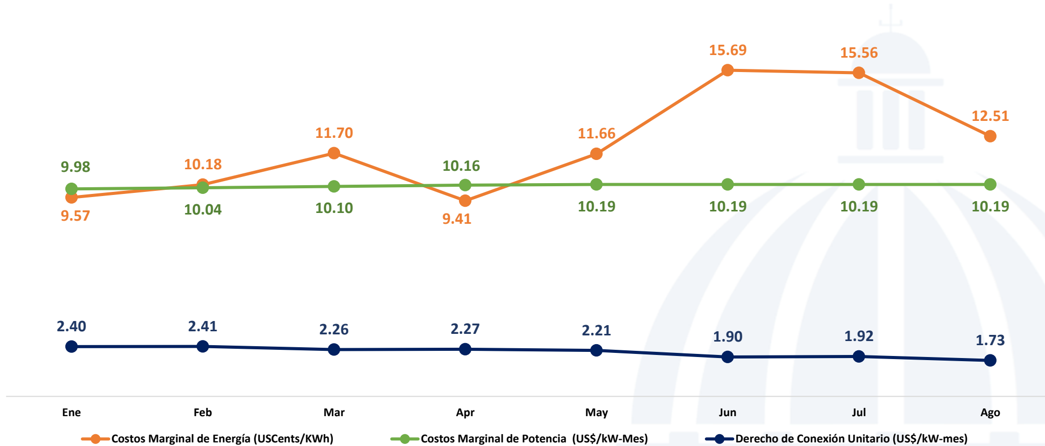
Costos Marginales de Energía, Potencia y Derecho de Conexión Unitario enero-agosto 2024 (USCents/kWh y US$/kW-período de)
