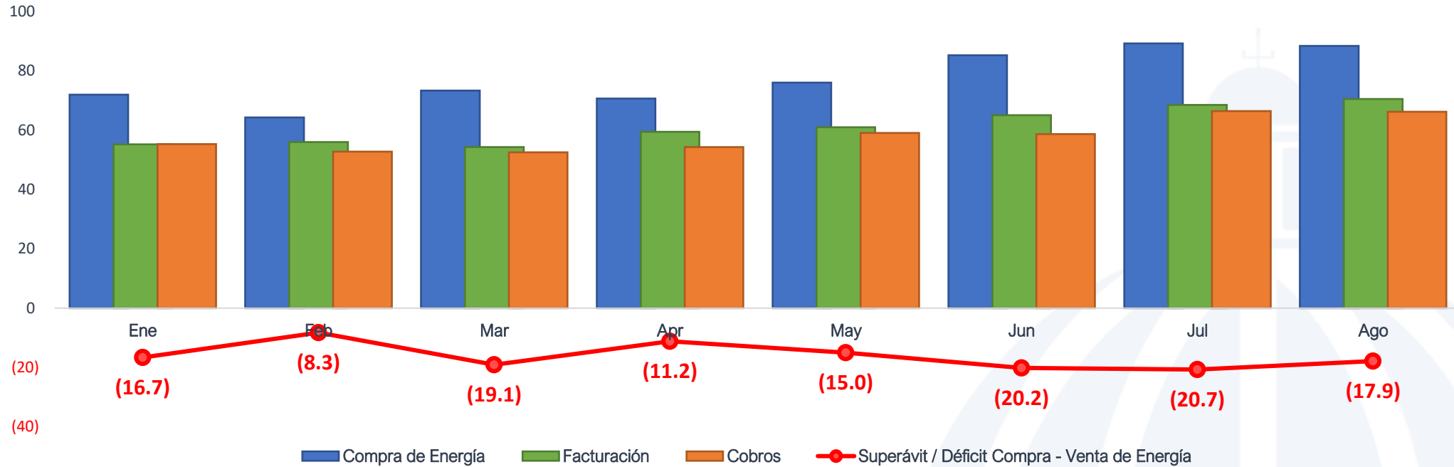
Factura de Compra - Facturación - Cobros Edenorte enero-agosto 2024 (US$ MM)
