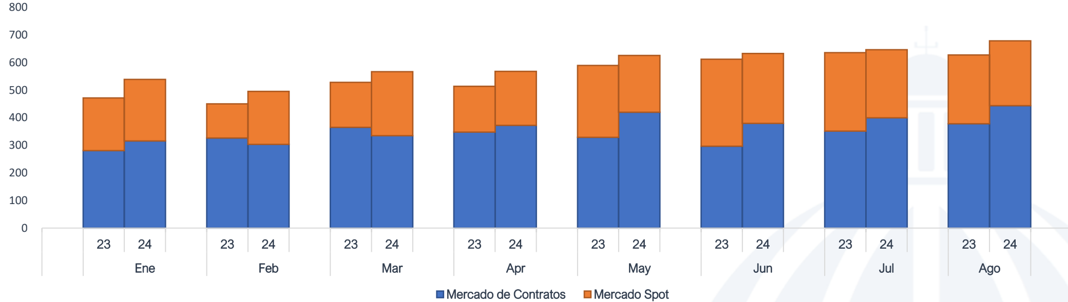
Compra de Energía por Mercado Edesur enero-agosto 2024/ enero-agosto 2023 (GWh)
