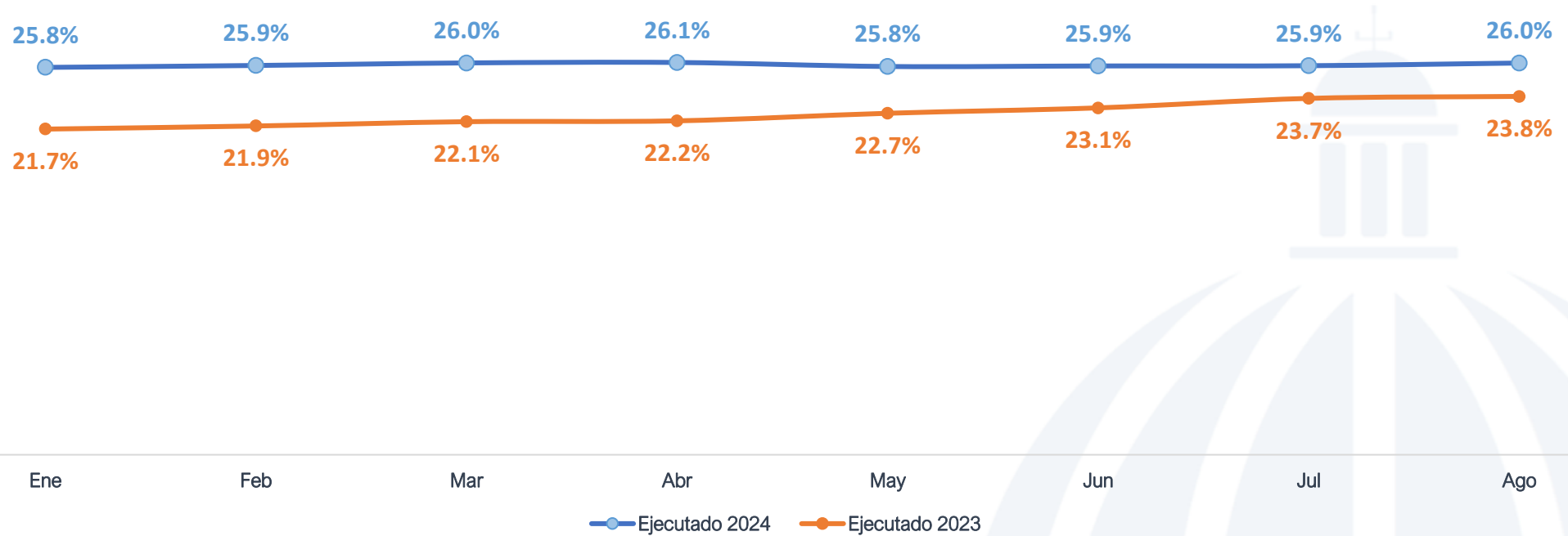
Pérdidas - Año Móvil Edenorte 2024 – 2023 Valores Porcentuales
