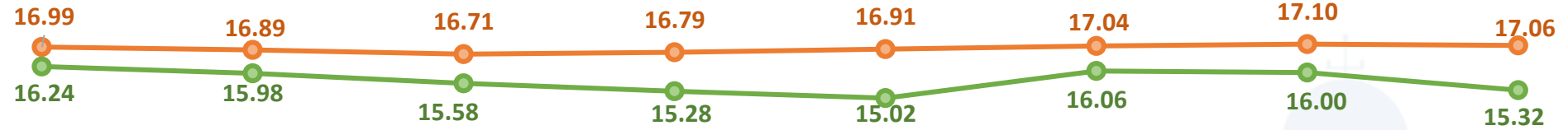
Precio Medio de Compra y Venta de Energía Edenorte enero-agosto 2024 (USCents/kWh)
