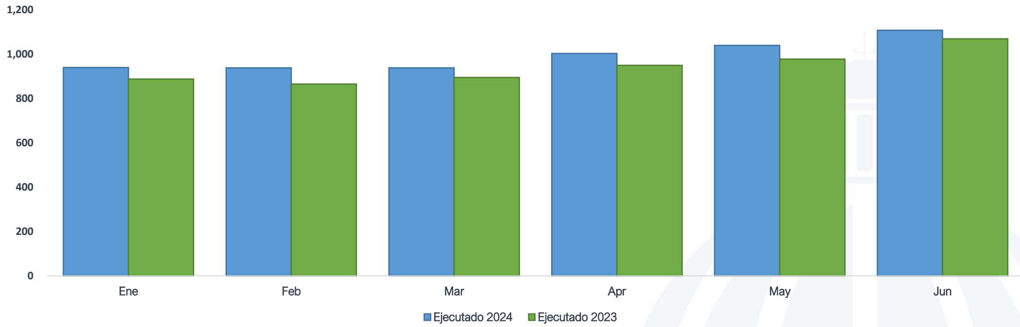
Energía Facturada Total EDE's enero-junio 2024/ enero-junio 2023 (GWh)
