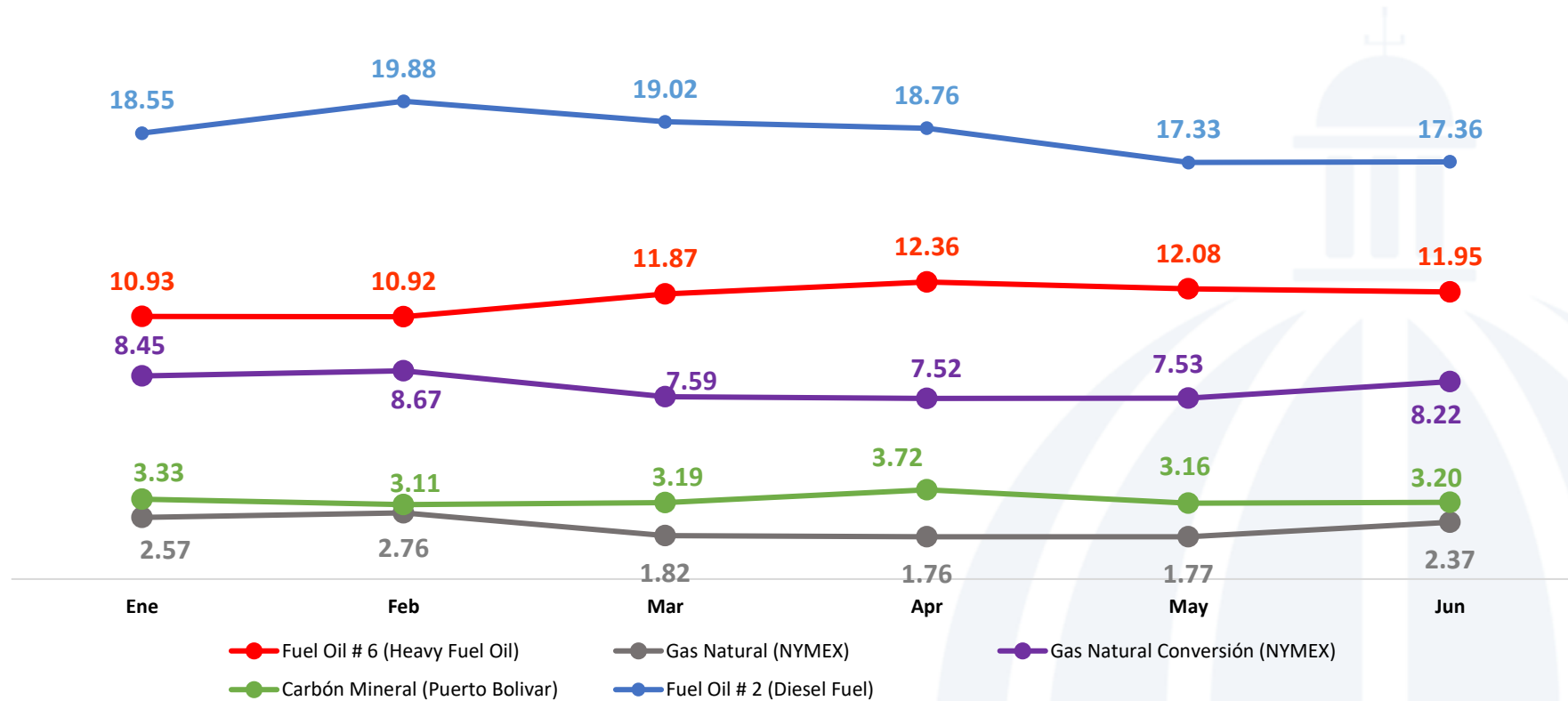
Precio de Combustibles enero-junio 2024 (US$/MMBTU)
