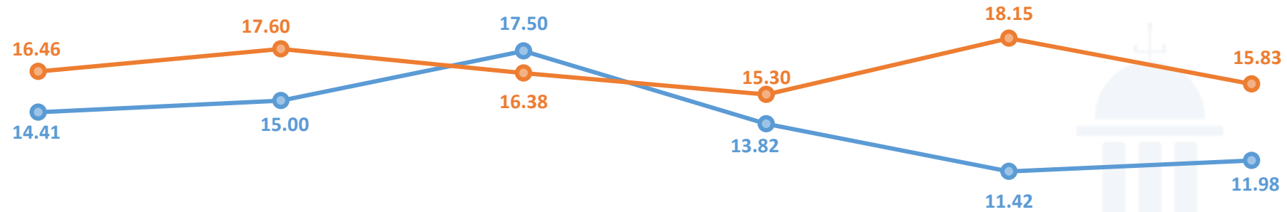
Precio Medio de Venta de Energía EGEHID enero-junio 2024/ enero-junio 2023 (USCents/kWh)
