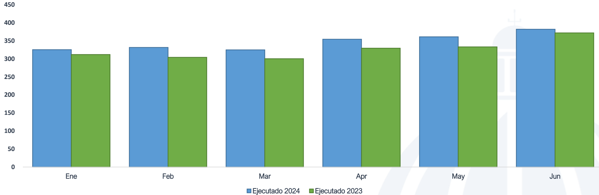
Energía Facturada Edenorte enero-junio 2024/ enero-junio 2023 (GWh)
