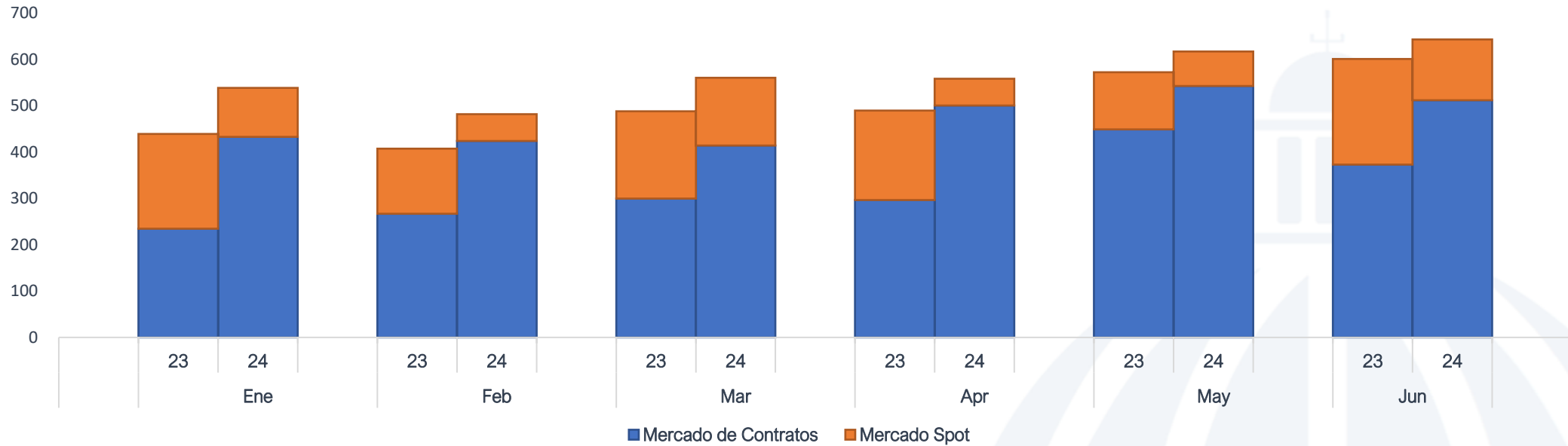
Compra de Energía por Mercado Edeeste enero-junio 2024- enero-junio 2023 (GWh)
