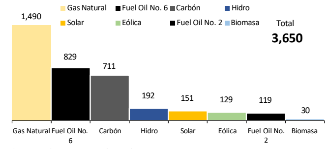
Disponibilidad promedio del SENI por combustible - junio 2024
