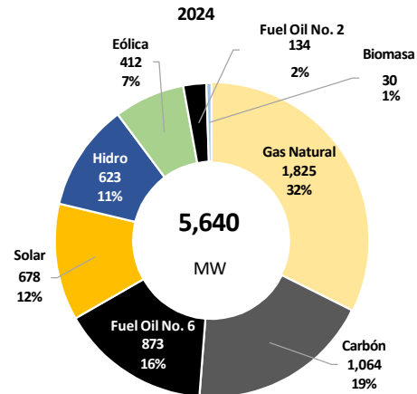
Matriz de capacidad nominal instalada - mayo 2024
