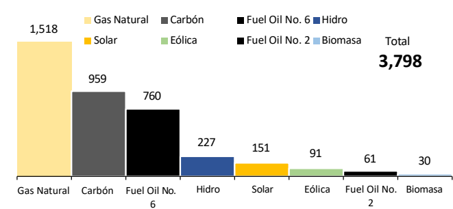
Disponibilidad promedio del SENI por combustible - mayo 2024
