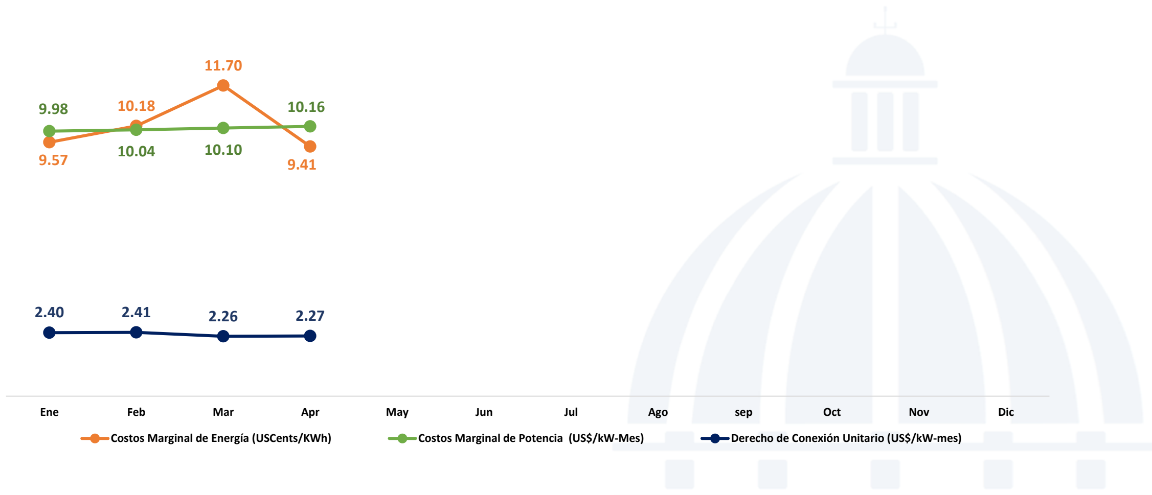
Costos Marginales de Energía, Potencia y Derecho de Conexión Unitario enero-abril 2024 (USCents/kWh y US$/kW-período de)
