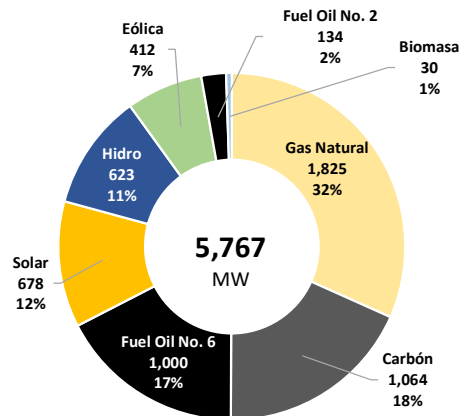
Matriz de capacidad nominal instalada - 2023
