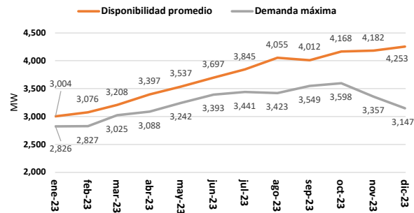
Evolución Disponibilidad promedio Centrales del SENI vs Demanda Máxima
