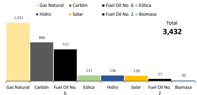
Disponibilidad promedio del SENI por combustible - 2023
