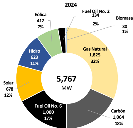
Matriz de capacidad nominal instalada - enero 2024
