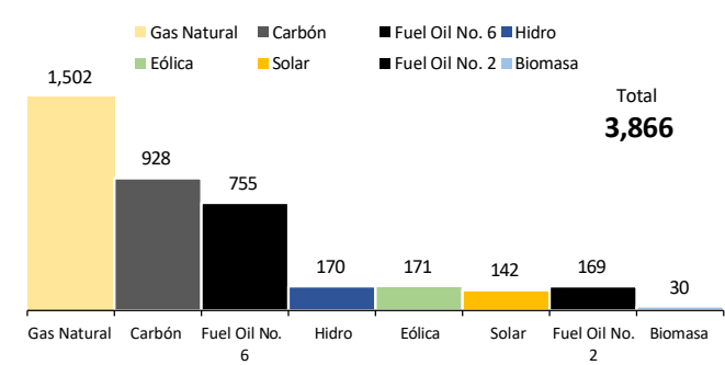
Disponibilidad del SENI por combustible - enero 2024
