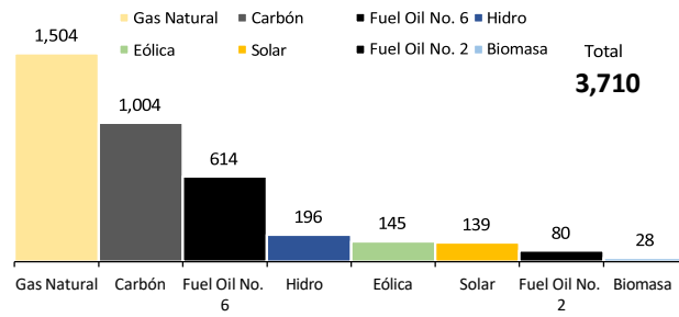
Disponibilidad del SENI por combustible - noviembre 2023
