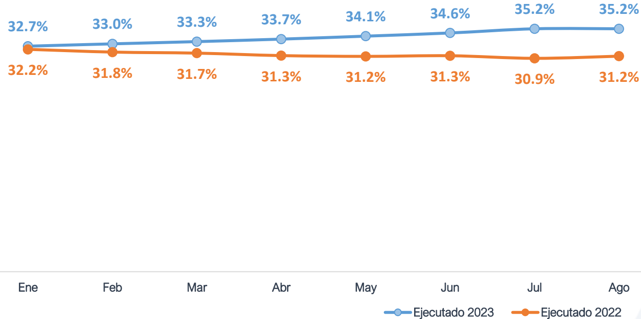
Pérdidas - Año Móvil Total EDE's 2023 - 2022 Valores Porcentuales
