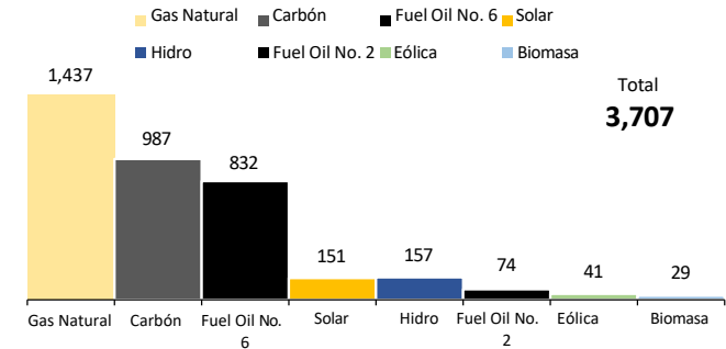
Disponibilidad del SENI por combustible - octubre 2023
