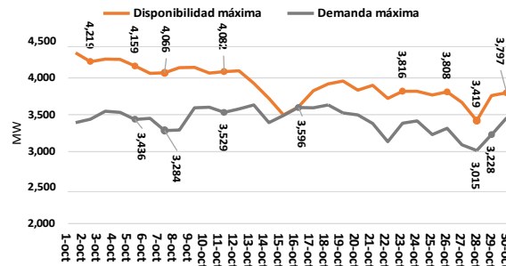
Evolución Disponibilidad Centrales del SENI vs Demanda Máxima
