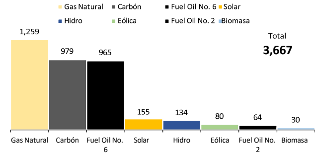
Disponibilidad del SENI por combustible - septiembre 2023
