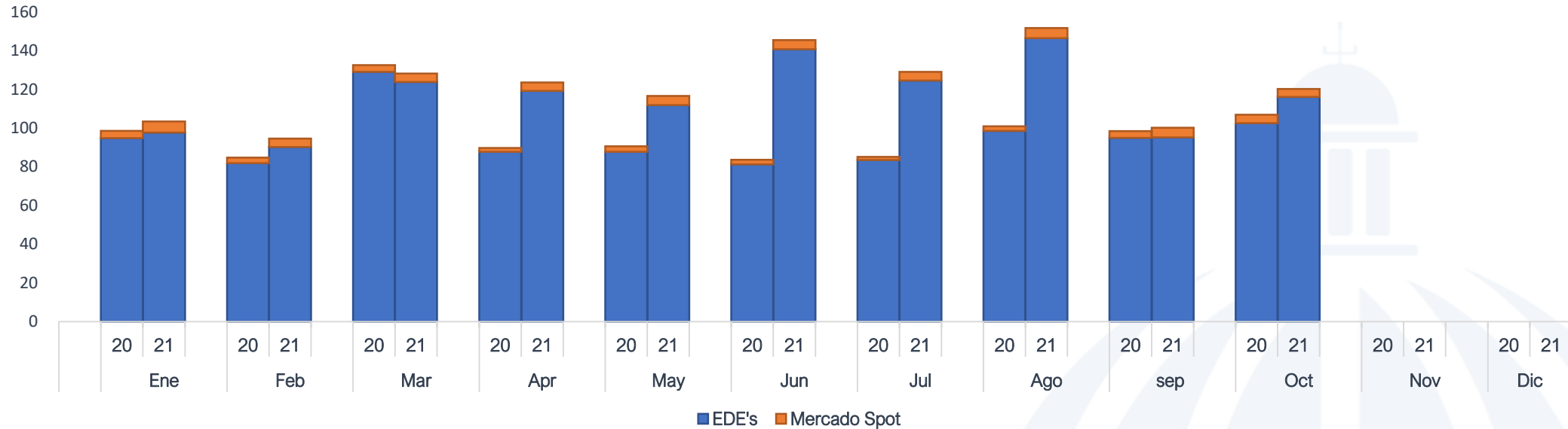
Energía Facturada EGEHID ene-oct 2021 / ene-oct 2020 (GWh)
