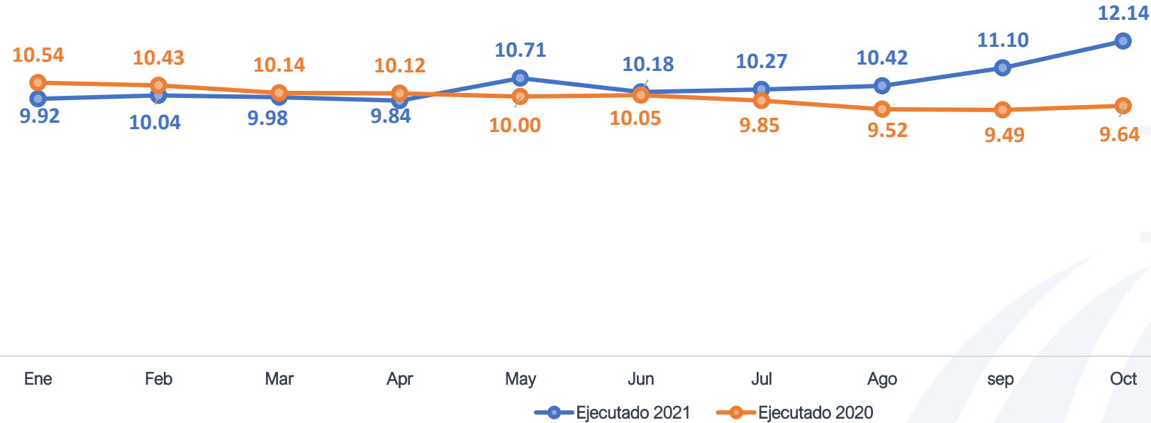
Precio Medio de Compra de Energía CDEEE ene-oct 2021 / ene-oct 2020 (USCents/kWh)
