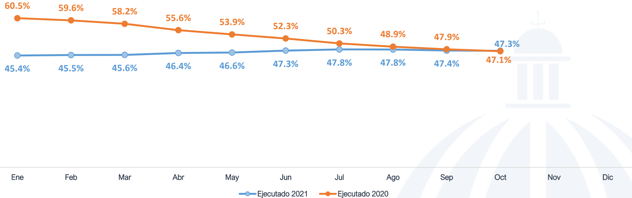
Índice de Recuperación de Energía - Año Móvil Edeeste 2021 – 2020 Valores Porcentuales
