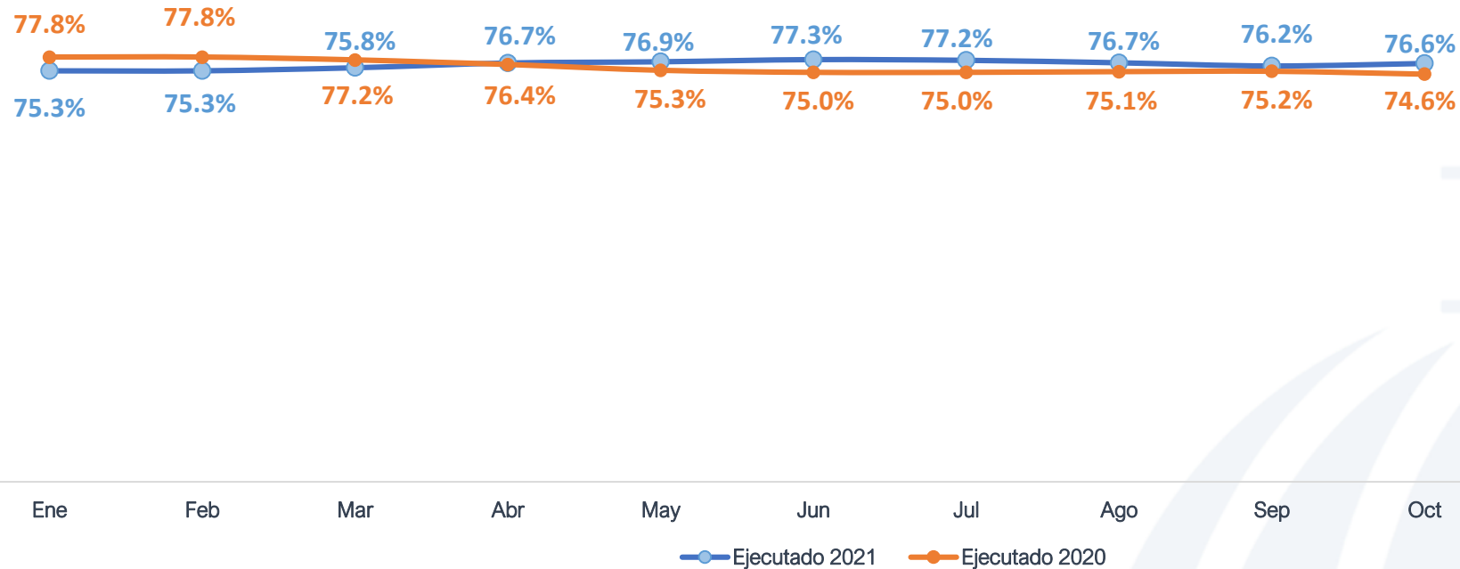
Índice de Recuperación de Energía - Año Móvil Edenorte 2021 – 2020 Valores Porcentuales
