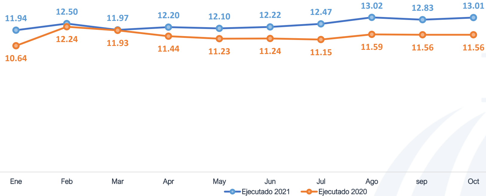
Precio Medio de Compra de Energía Edenorte ene-oct 2021 / ene-oct 2020 (USCents/kWh)
