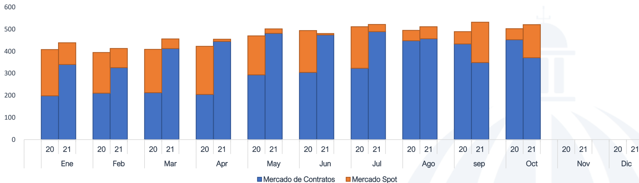
Compra de Energía por Mercado Edeeste ene-oct 2021 / ene-oct 2020 (GWh)
