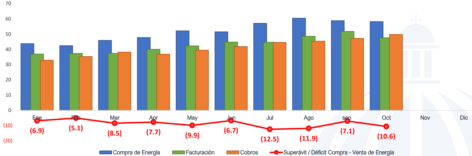
Factura de Compra - Facturación - Cobros Edenorte ene-oct 2021 (US$ MM)
