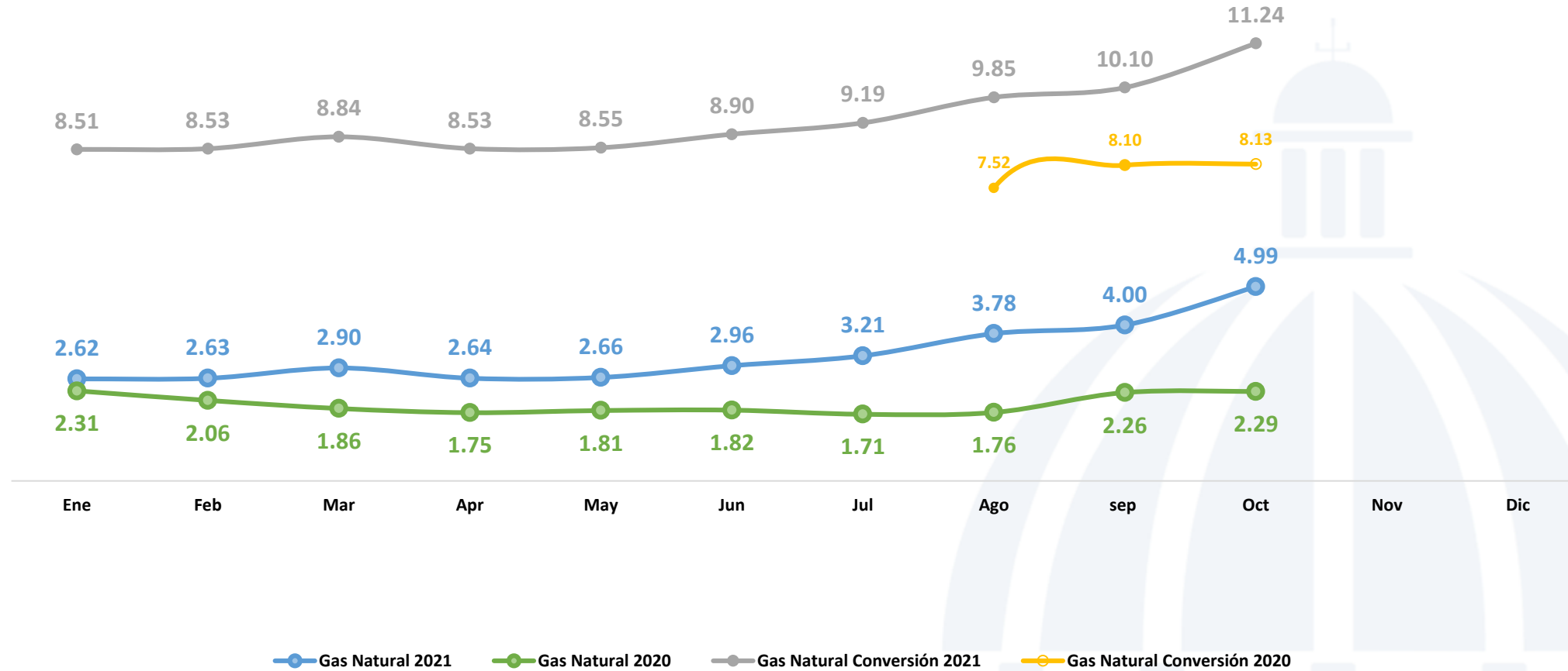
Precio de Combustible Gas Natural ene-oct 2021 / ene-oct 2020 (US$/MMBTU)
