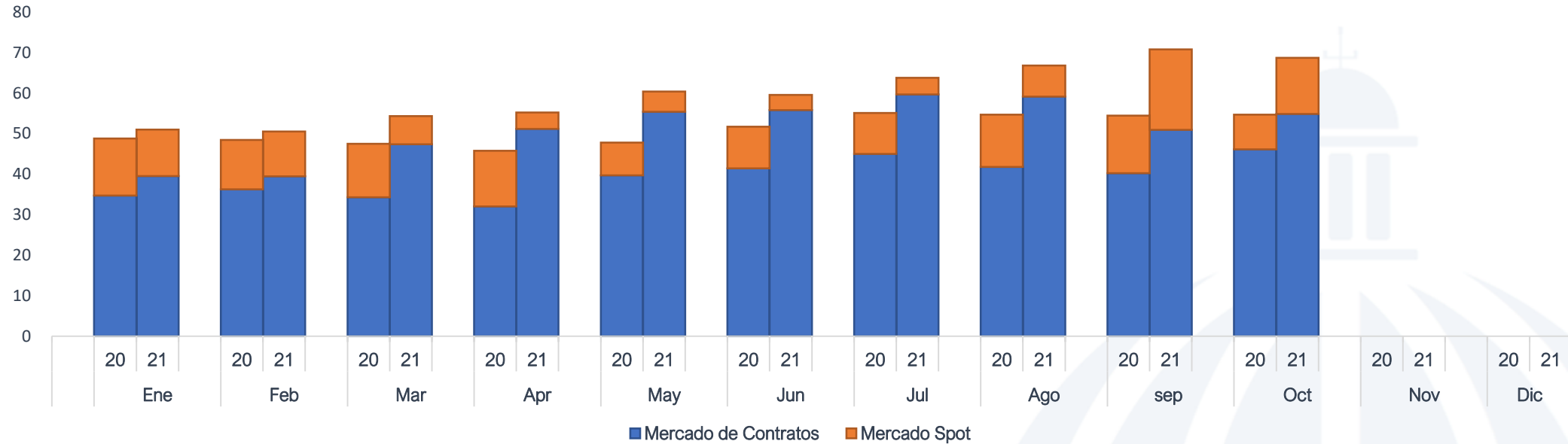
Factura Compra de Energía por Mercado Edesur ene-oct 2021 / ene-oct 2020 (US$ MM)
