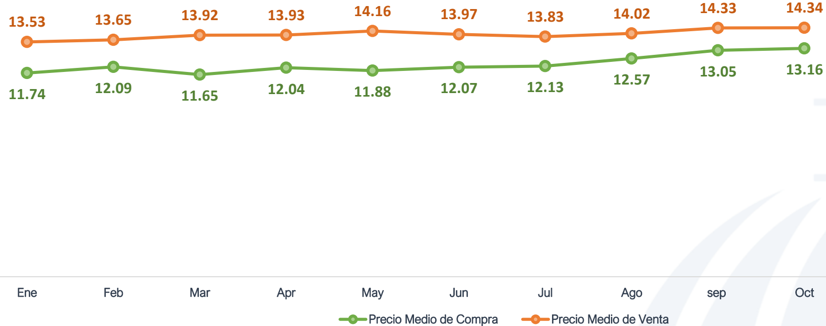
Precio Medio de Compra y Venta de Energía Total EDE's ene-oct 2021 (USCents/kWh)
