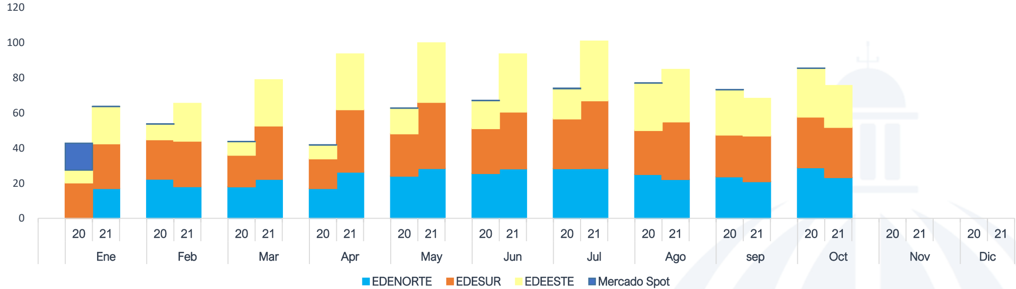
Factura por Venta de Energía CDEEE ene-oct 2021 / ene-oct 2020 (US$ MM)
