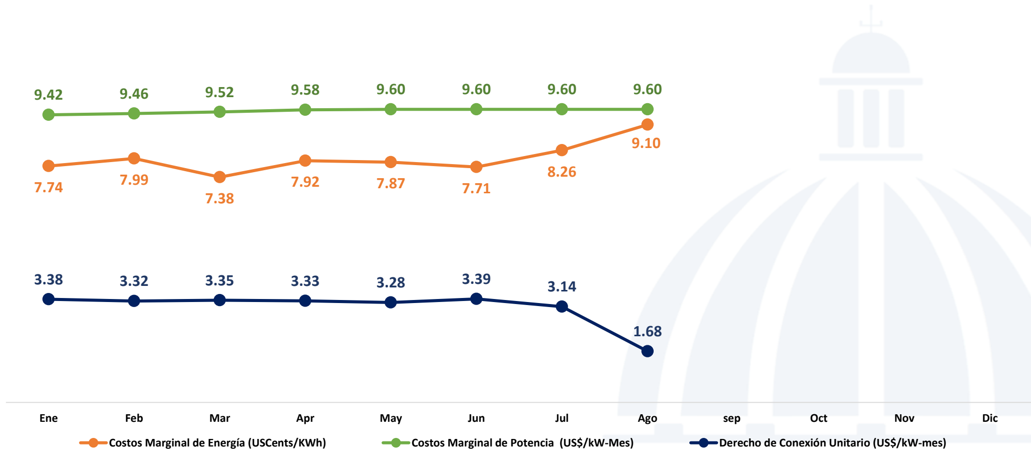
Costos Marginales de Energía, Potencia y Derecho de Conexión Unitario ene-ago 2021 (USCents/kWh y US$/kW-Mes)
