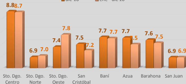
Monómico EDESur (RD$/kWh)
