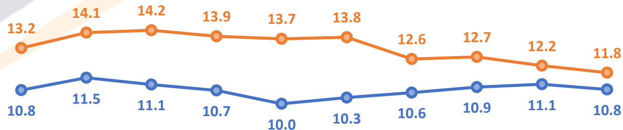
Precio Medio de Compra de Energía Total EDE's Ene-Oct 2020 – Ene-Oct 2019 USCents/kWh
