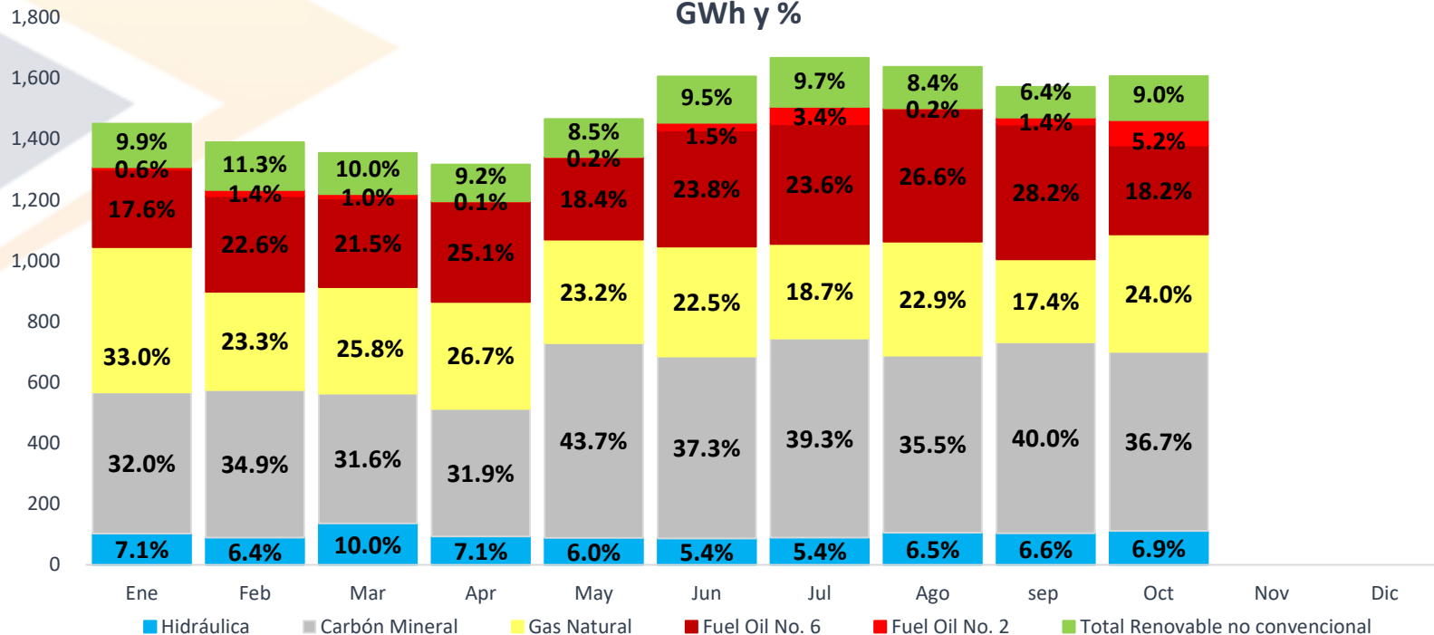
Generación de Energía por Tipo de Combustible Enero- Oct 2020 GWh y %
