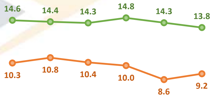
Precio Medio de Compra y Venta de Energía Edeeste Enero - Diciembre 2020 USCents/kWh
