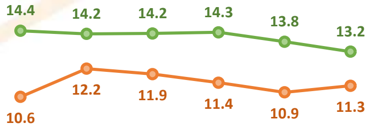
Precio Medio de Compra y Venta de Energía Edenorte Enero - Diciembre 2020 USCents/kWh
