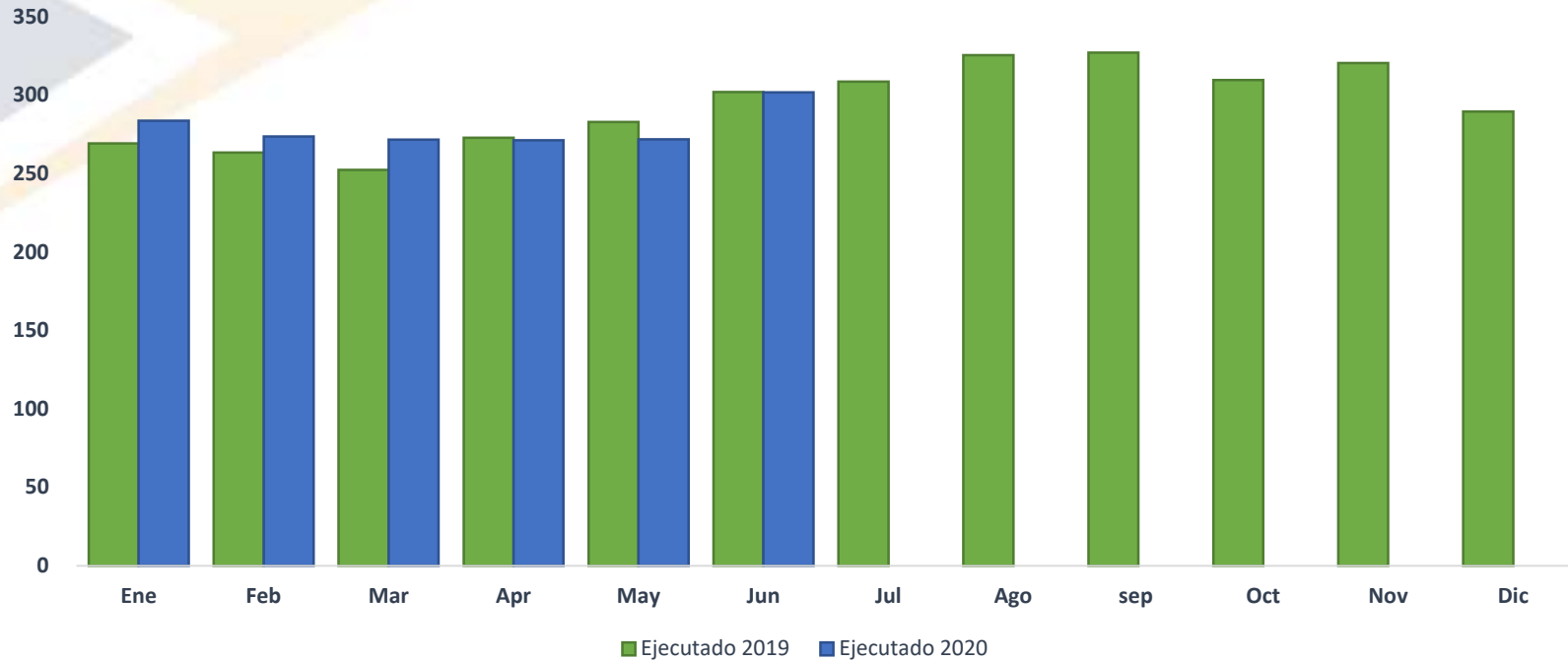
Energía Facturada Edenorte 2020 - 2019 GWh
