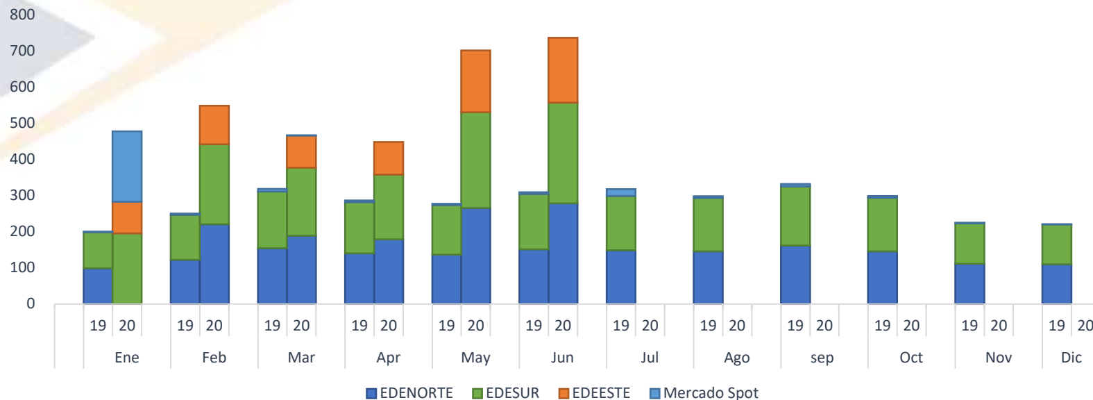
Energía Facturada CDEEE 2020 - 2019 GWh
