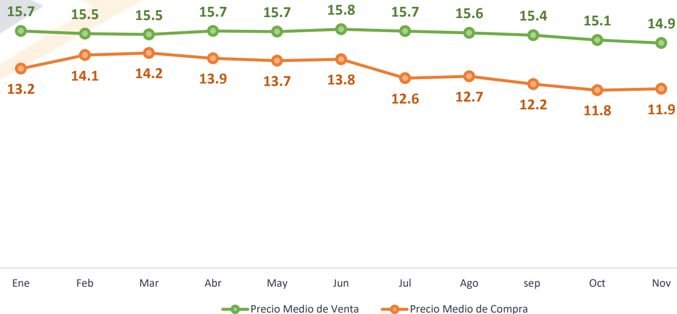
Precio Medio de Compra y Venta de Energía Total EDE's Enero- Diciembre 2019 USCents/kWh
