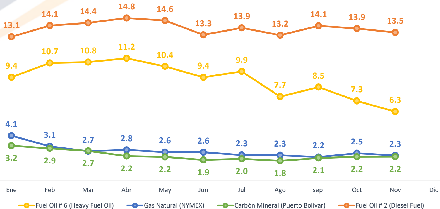
Precio de Combustibles 2019 US$/MMBTU
