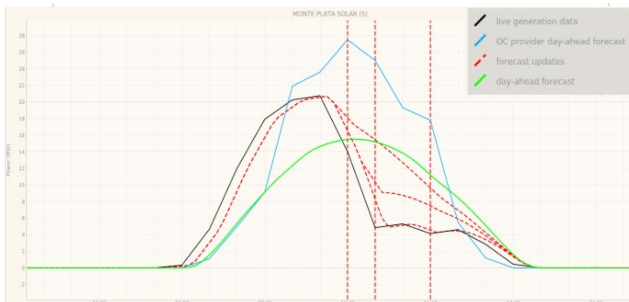
Figura 28. Pronóstico con optimización a corto plazo para Monte Plata Solar
