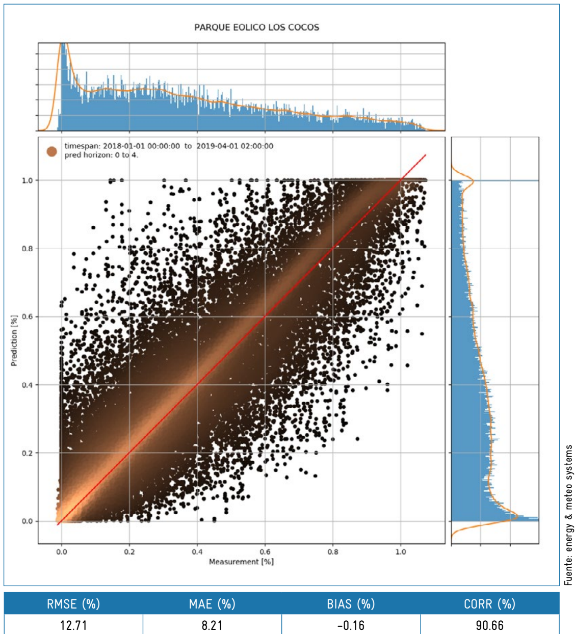
Figura 19. emsys diagrama de dispersión para pronóstico intradía Los Cocos
