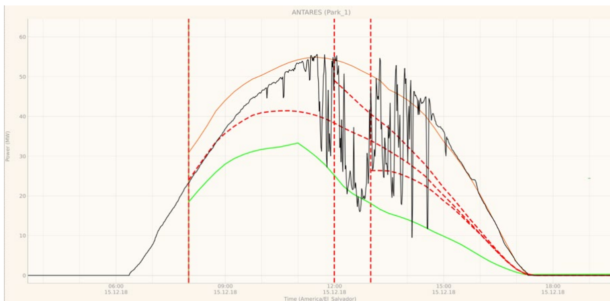
Figura 33. Spread (distribución) de pronóstico de potencia solar
