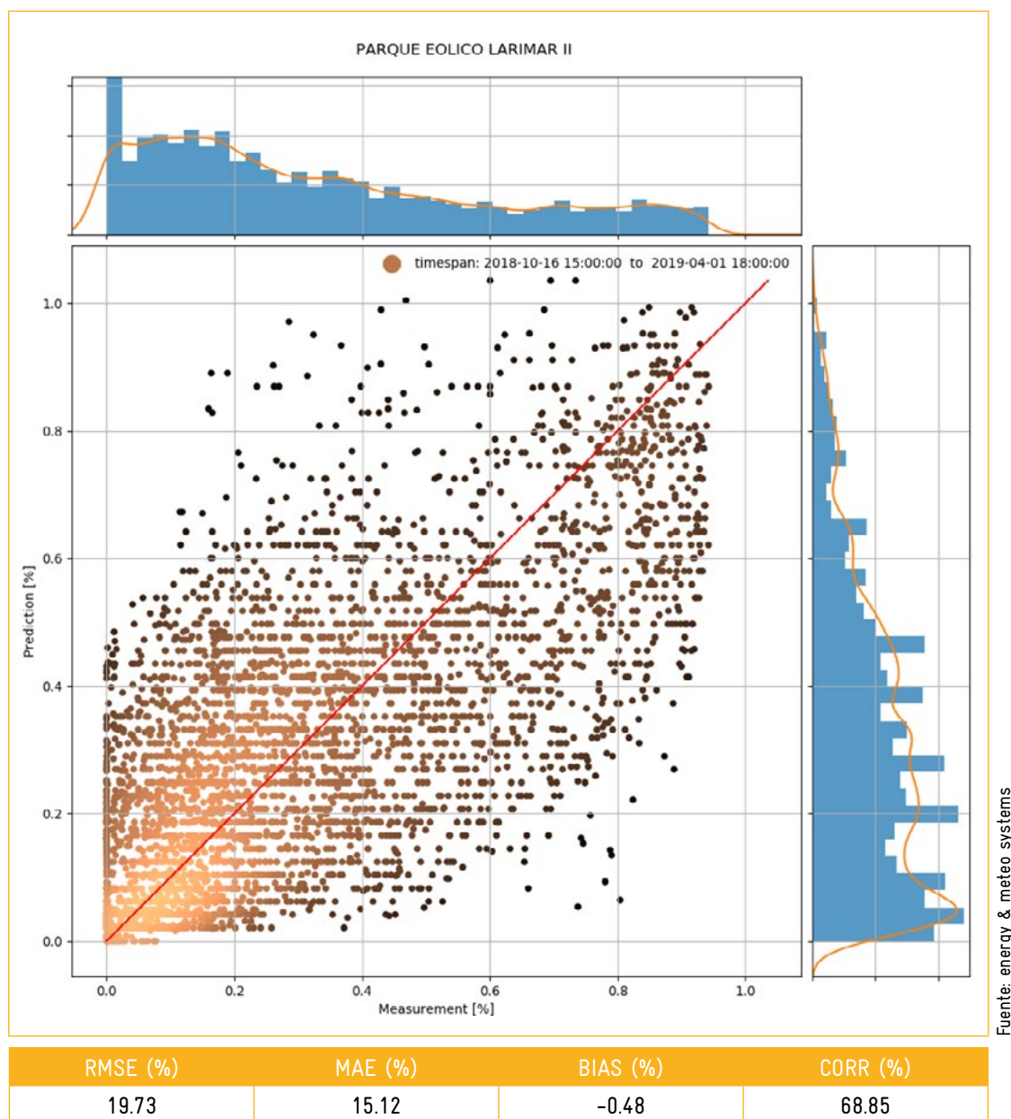
Figura 10. Diagrama de dispersión para pronóstico intradía Larimar II
