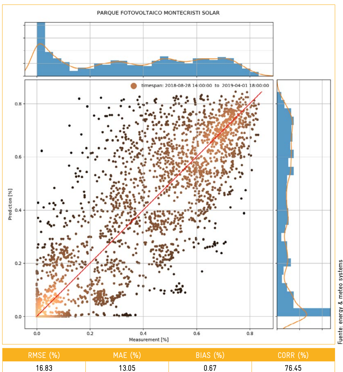
Figura 7. Diagrama de dispersión para pronóstico de día en adelante Montecristi Solar
