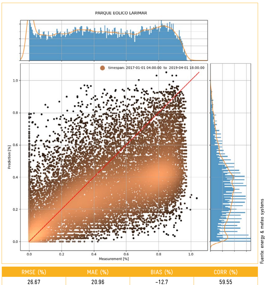
Figura 3. Diagrama de dispersión para pronóstico día en adelante Larimar I
