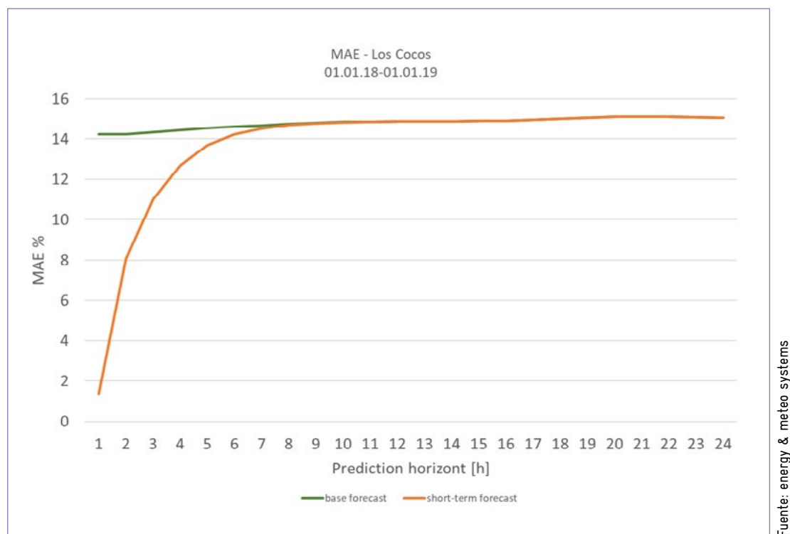
Figura 30. Comparación de MAE pronóstico base vs. optimización a corto plazo
