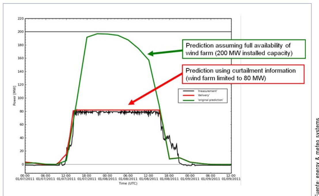
Figura 32. Planes de producción incluyendo no disponibilidades o recortes de potencia incluidos en el pronóstico. Fuente: energy & meteo systems
