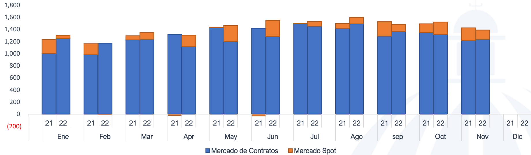
Compra de Energía por Mercado Total EDE's enero-noviembre 2022 / enero-noviembre 2021 (GWh)
