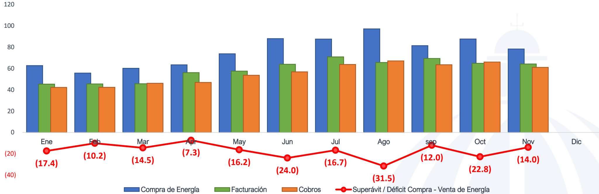
Factura de Compra - Facturación - Cobros Edenorte enero-noviembre 2022 (US$ MM)
