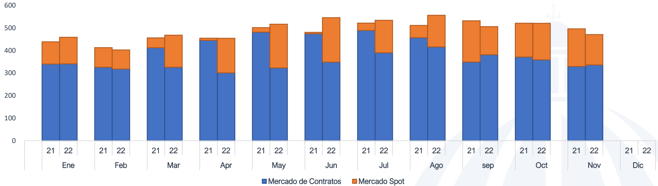
Compra de Energía por Mercado Edeeste enero-noviembre 2022 / enero-noviembre 2021 (GWh)
