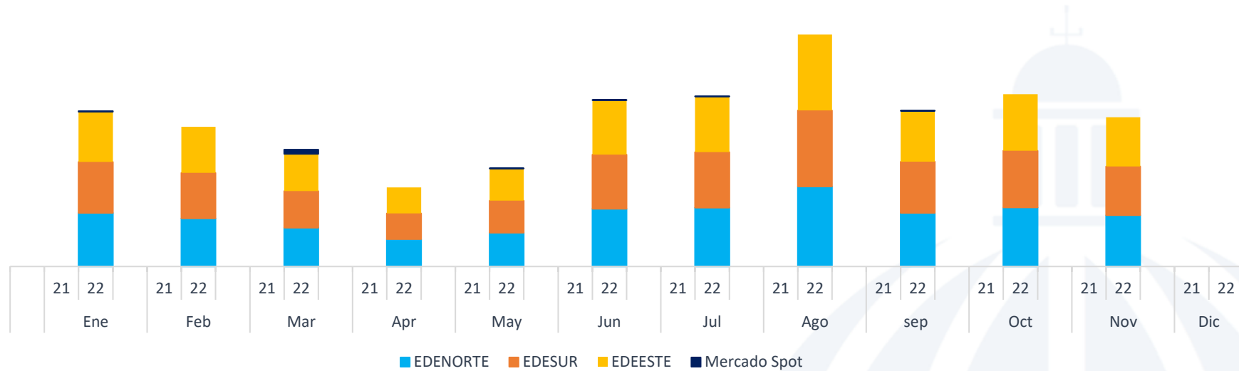
Factura por Venta de Energía Punta Catalina 2022 US$ MM
