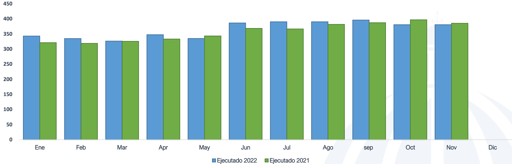
Energía Facturada Edesur enero-noviembre 2022 / enero-noviembre 2021 (GWh)
