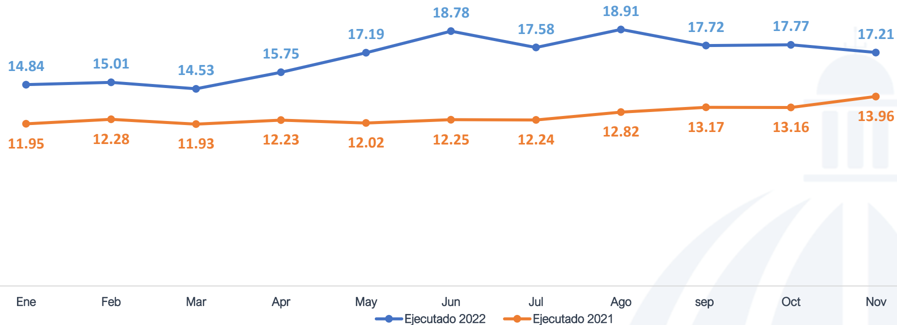
Precio Medio de Compra de Energía Edesur enero-noviembre 2022 / enero-noviembre 2021 (USCents/kWh)
