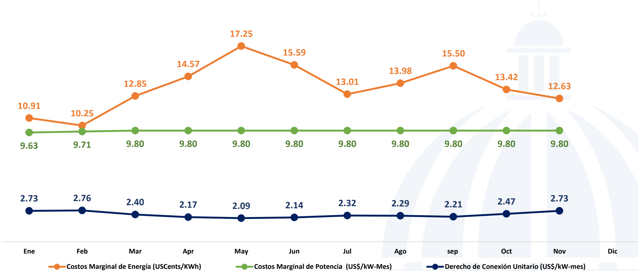
Costos Marginales de Energía, Potencia y Derecho de Conexión Unitario enero-noviembre 2022 (USCents/kWh y US$/kW-período)
