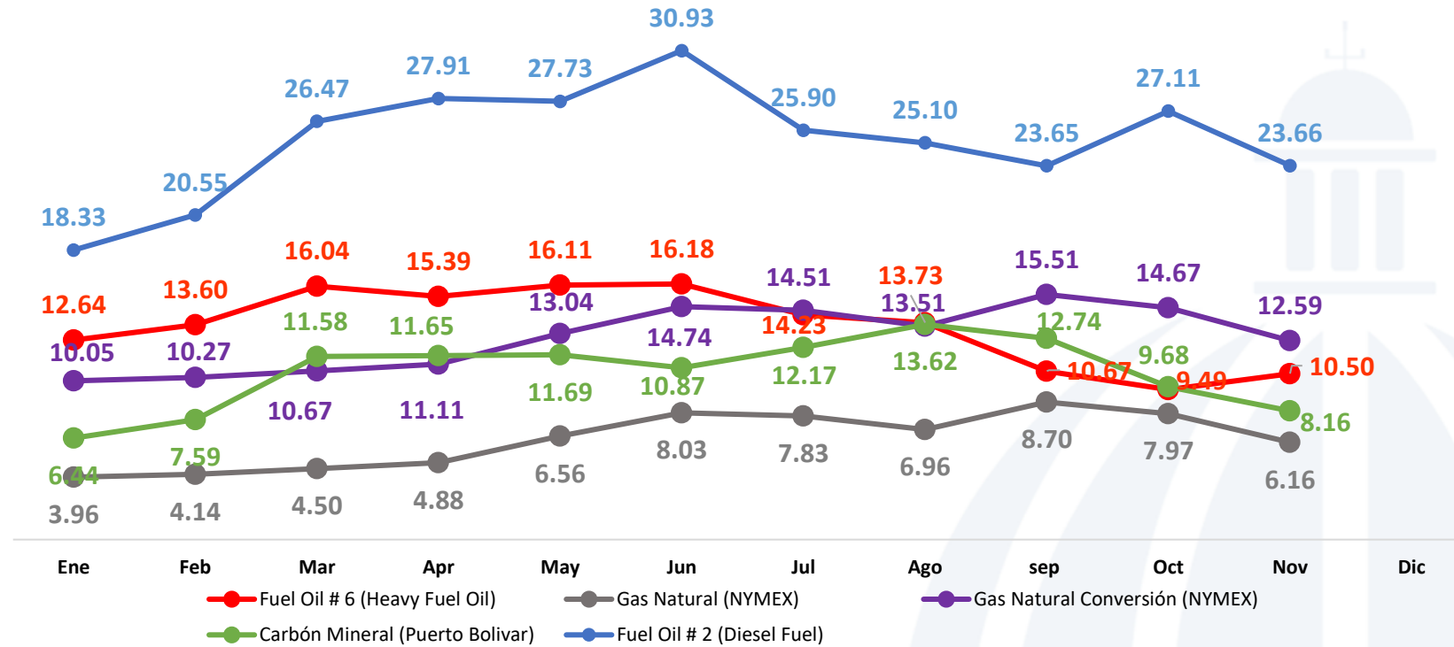
Precio de Combustibles enero-noviembre 2022 (US$/MMBTU)
