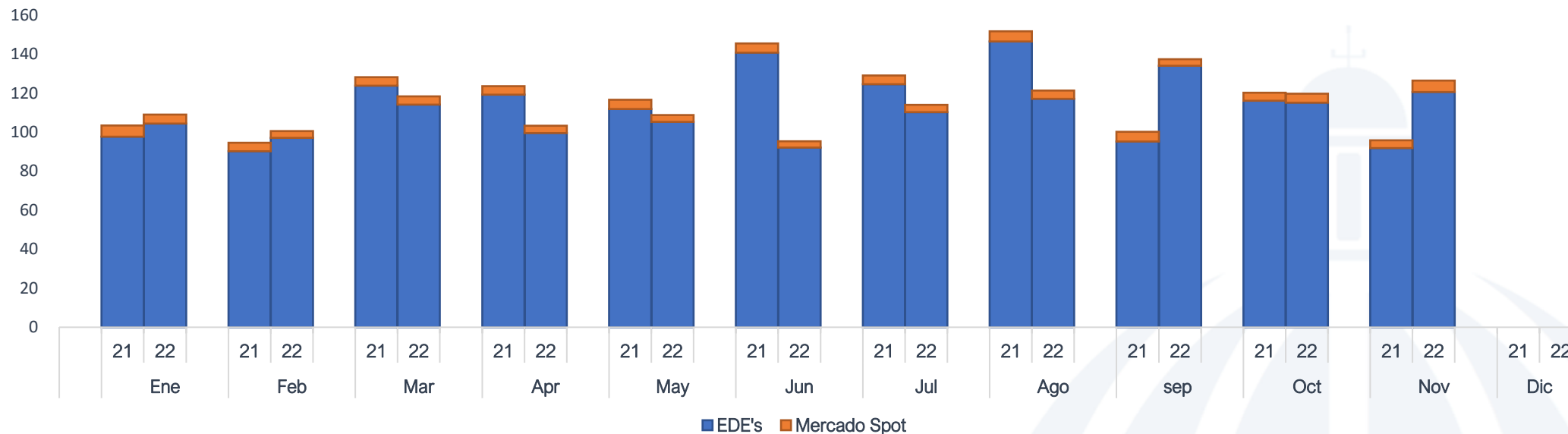
Energía Facturada EGEHID enero-noviembre 2022 / enero-noviembre 2021 (GWh)
