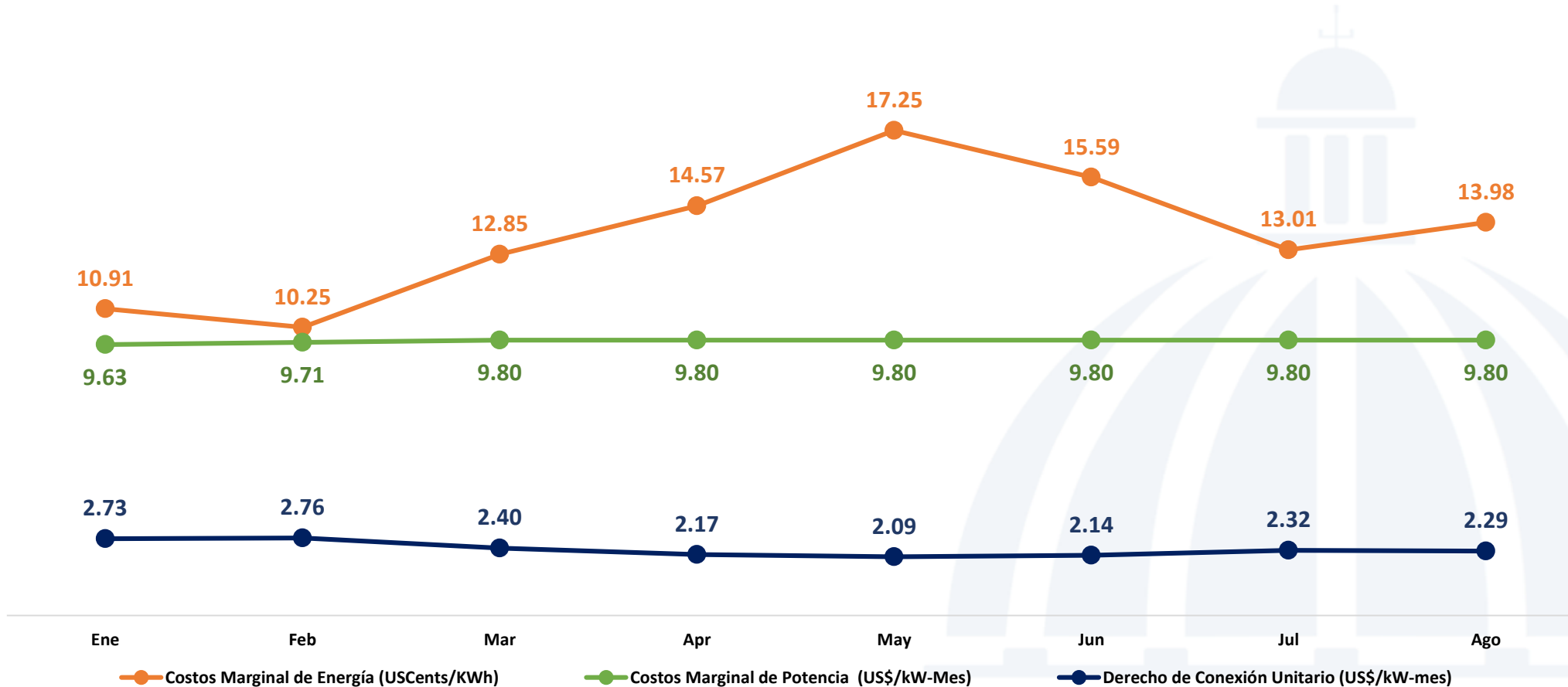
Costos Marginales de Energía, Potencia y Derecho de Conexión Unitario enero-agosto 2022 (USCents/kWh y US$/kW-período)
